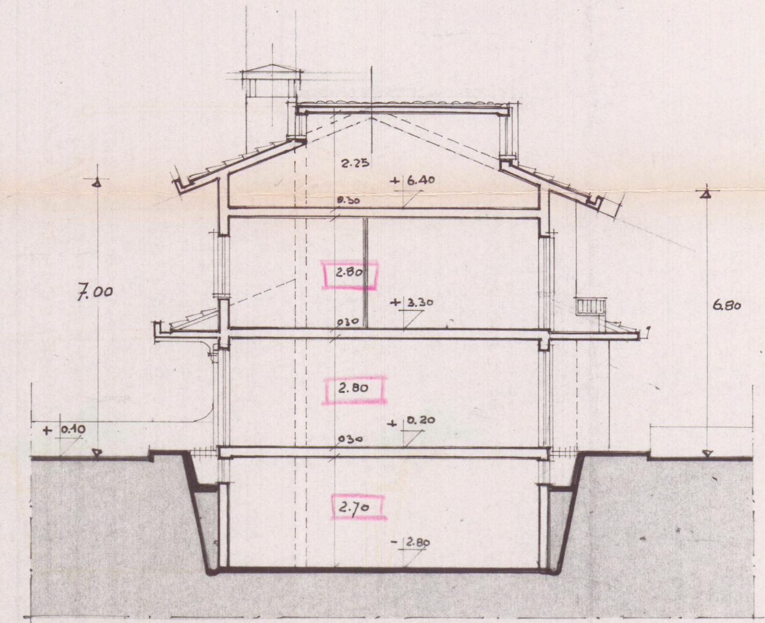
SEZIONE
