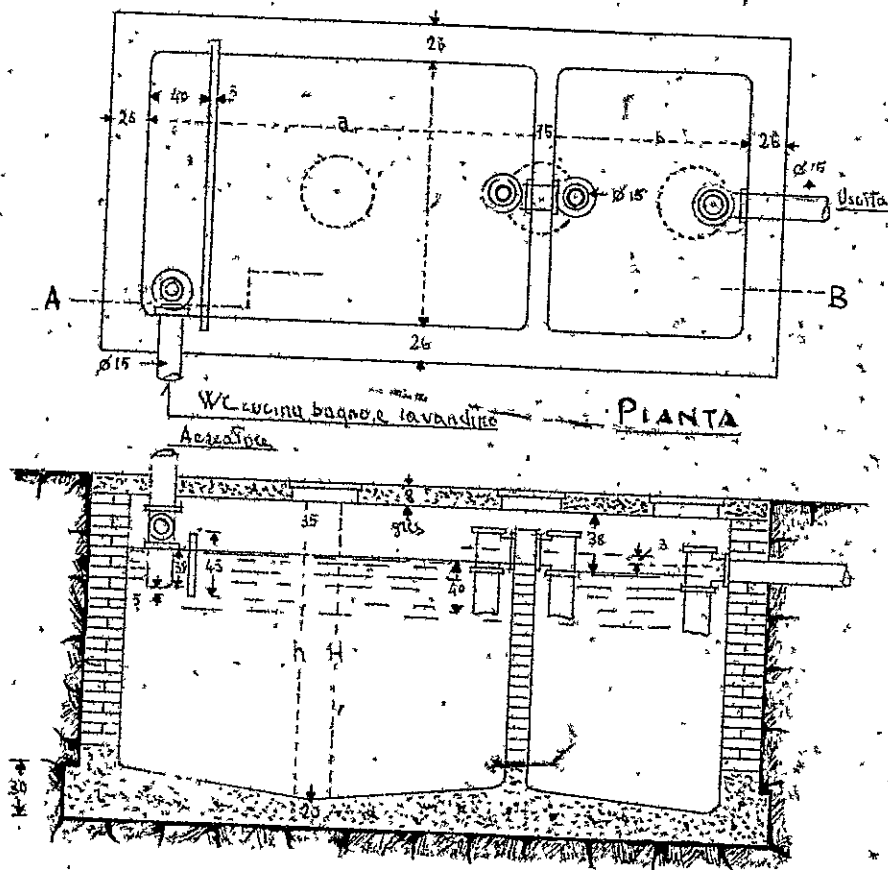
SEZIONE A-B
