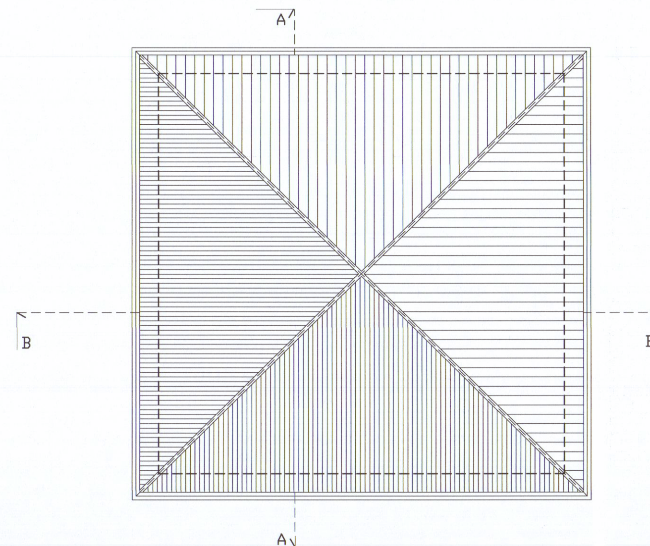
PIANTA COPERTURA
