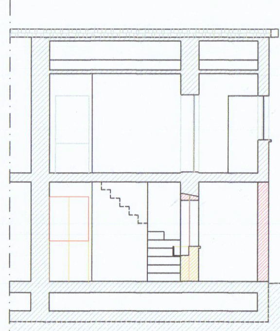
SEZIONE B-B' scala 1.100
