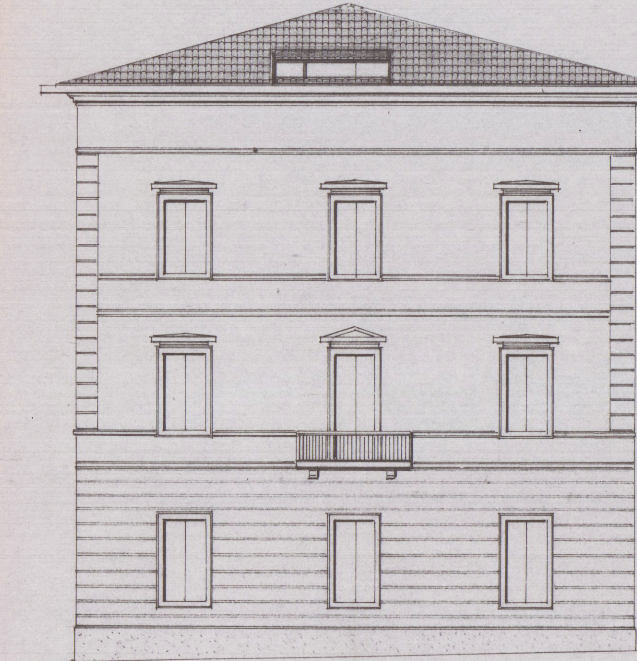
PROSPETTO SU V. BUONARROTI
