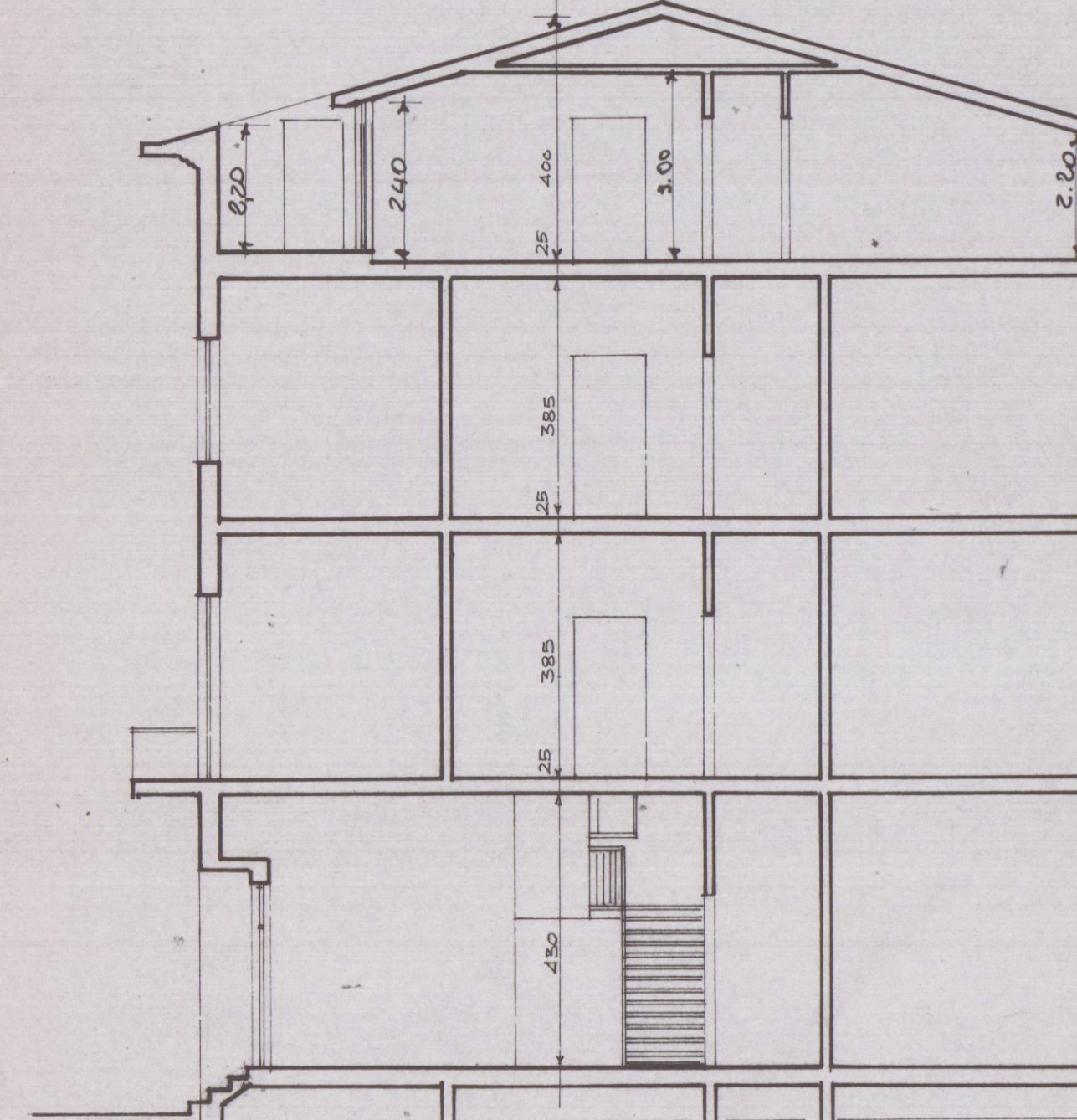
SEZIONE B-B'
