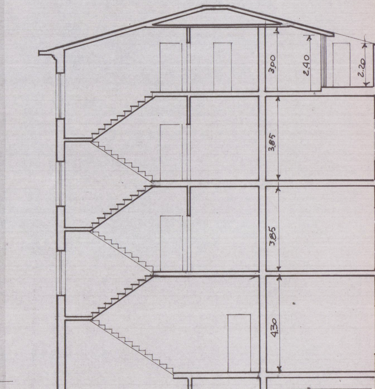
SEZIONE A-A'
