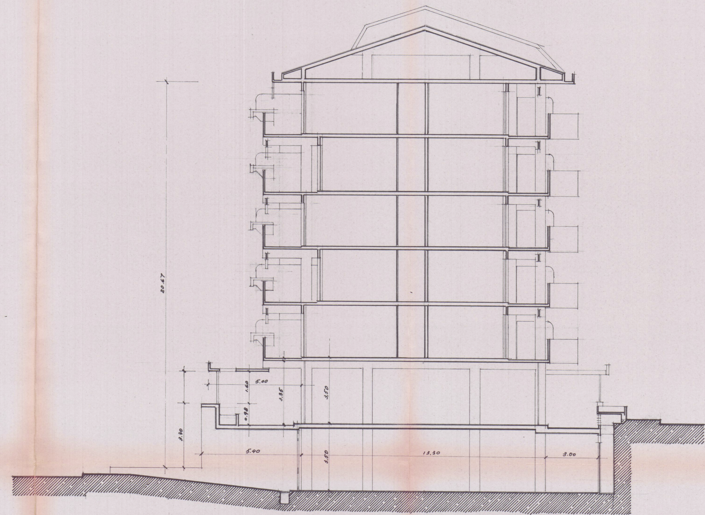
sezione CD
