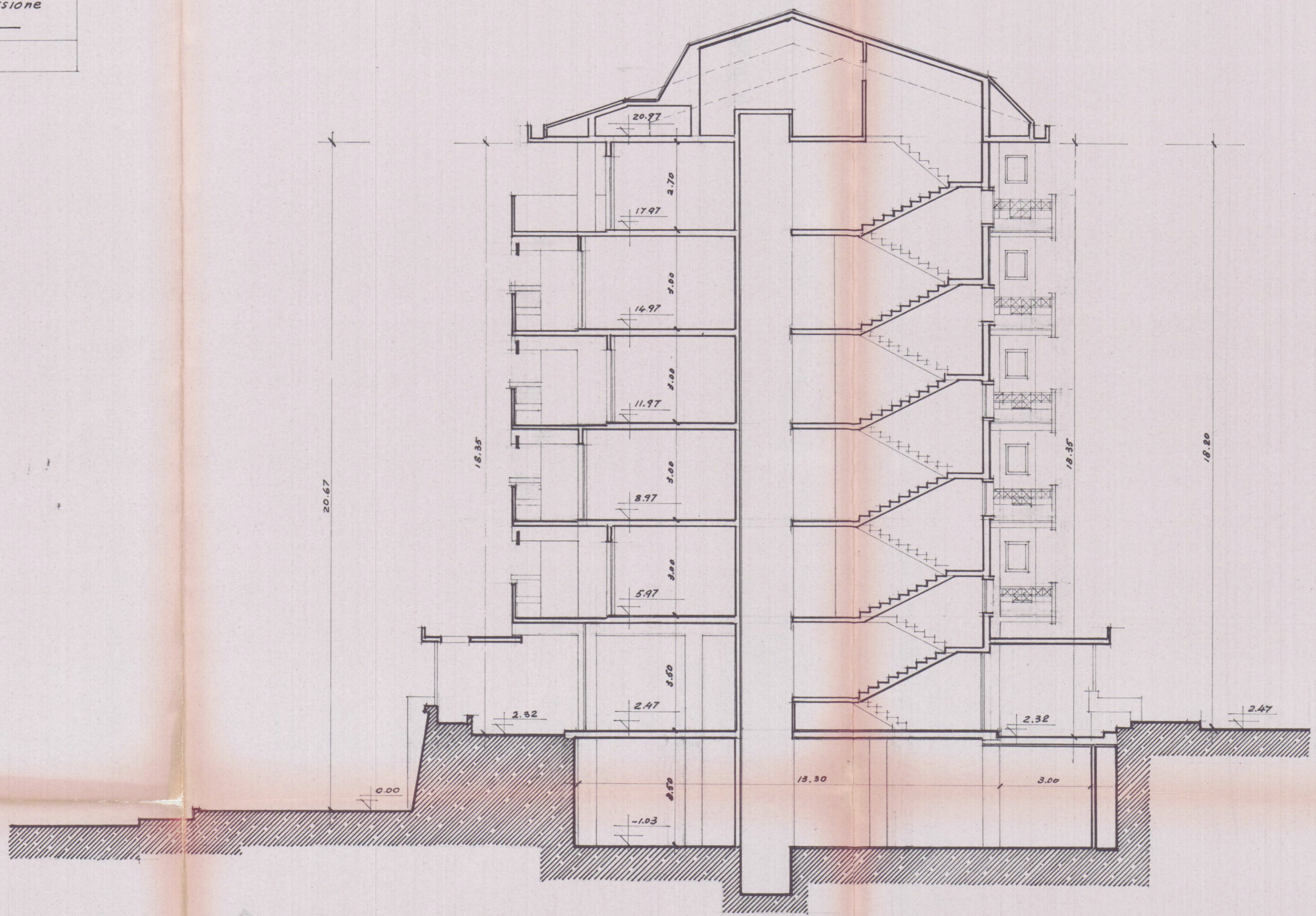
sezione AB
