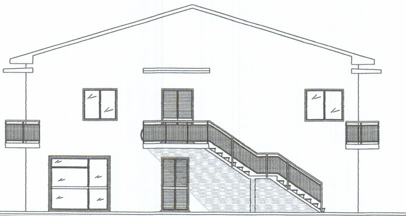
PROSPETTO OVEST
