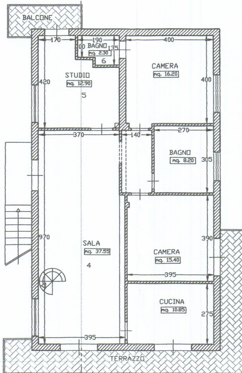
PIANO PRIMO
