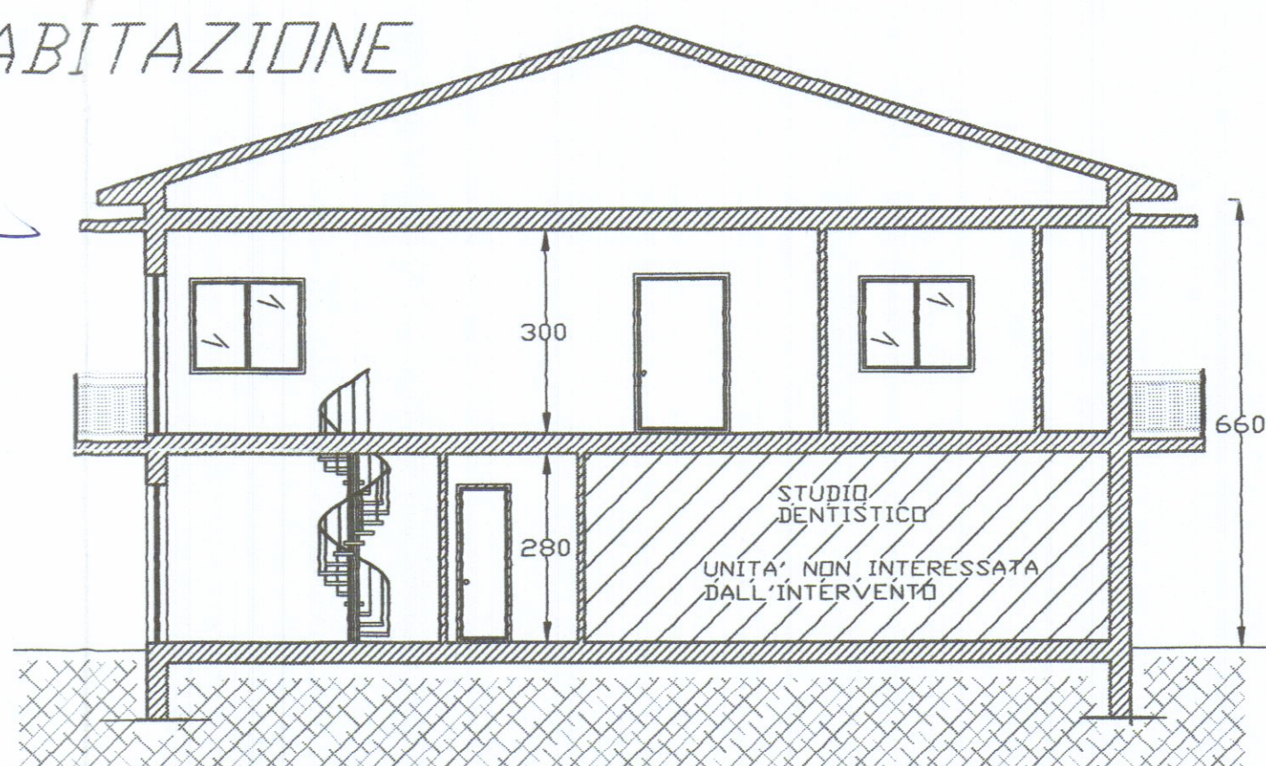
SEZIONE D-D
