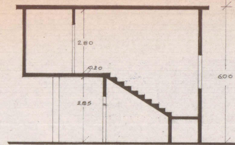
sezione A-A
