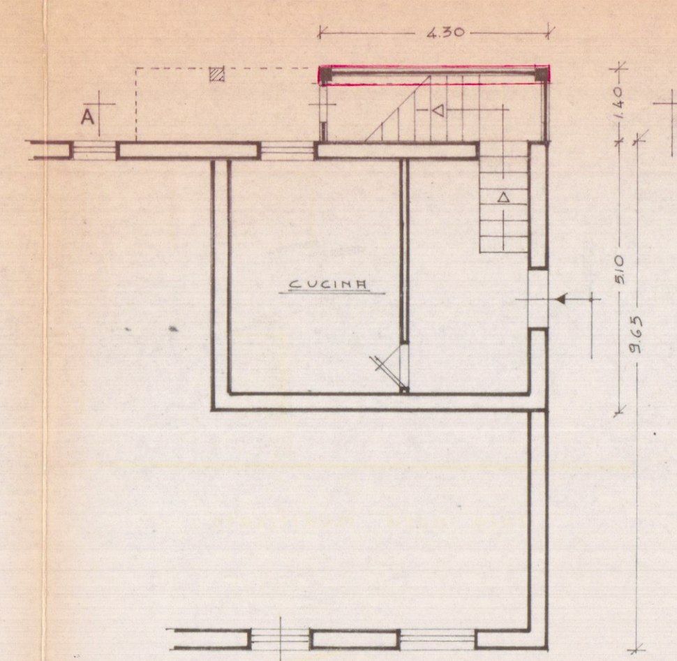
Piano terra modificato
