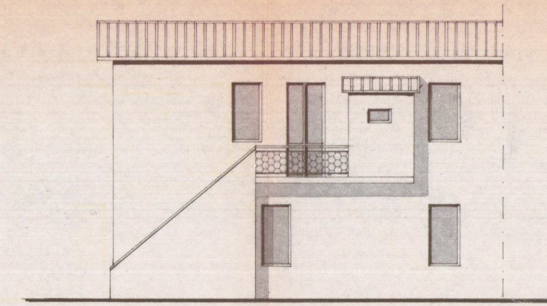
lato nord esistente
