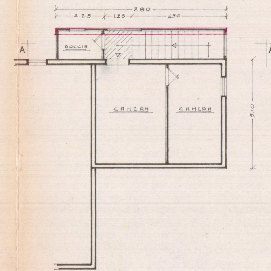
piano Primo modificato
