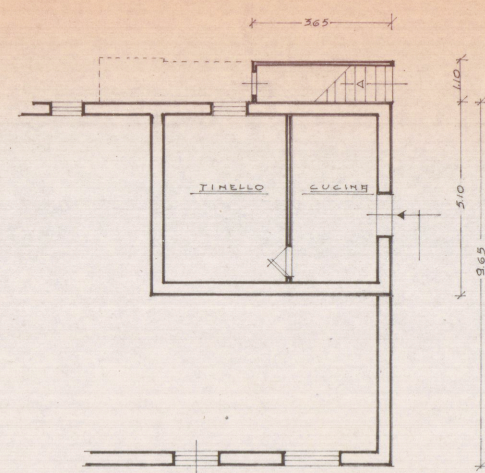
Piano terra esistente
