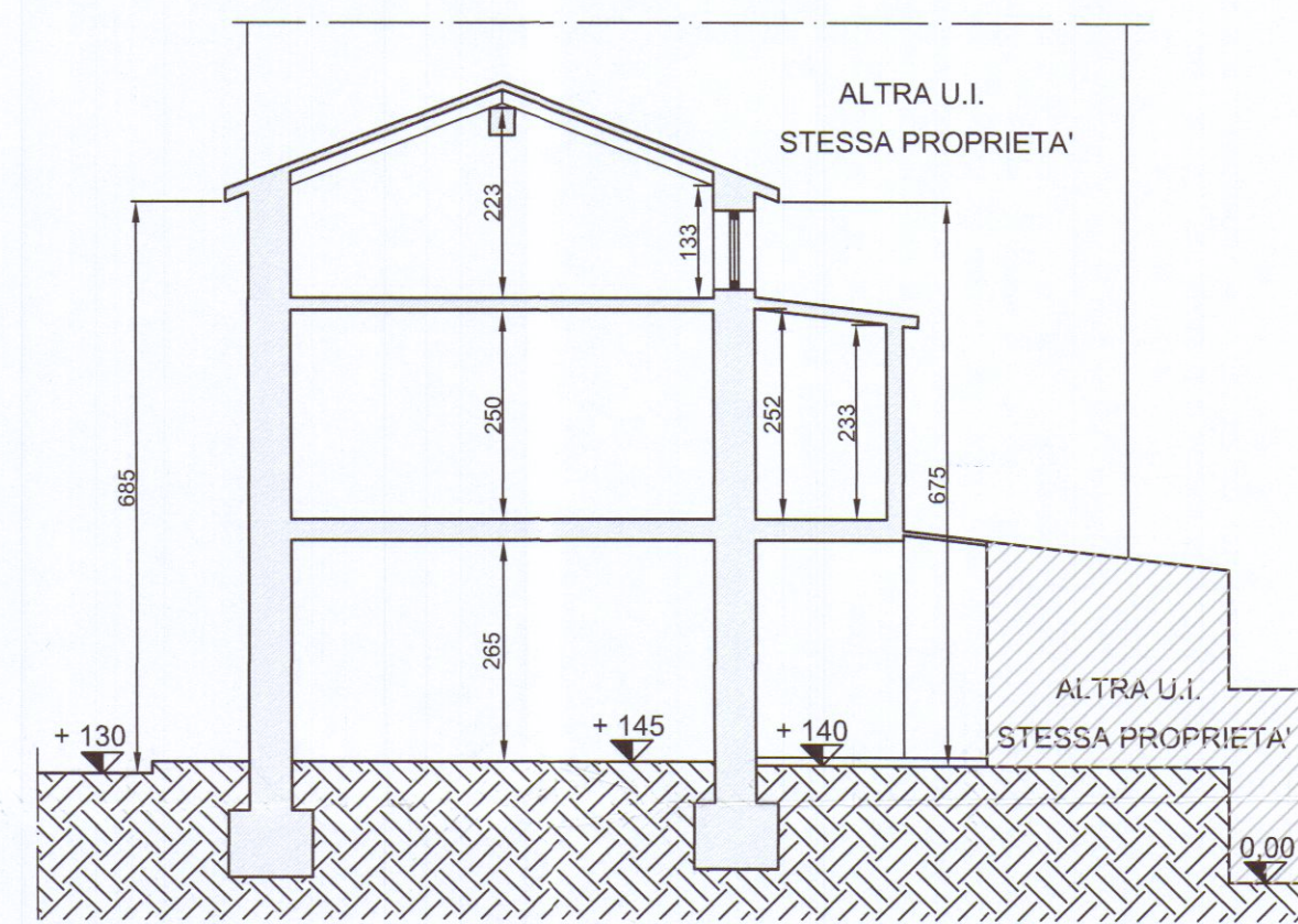
SEZIONE A-A
