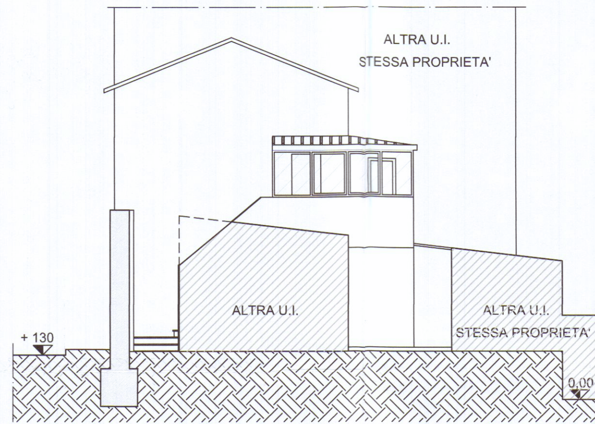
PROSPETTO OVEST
