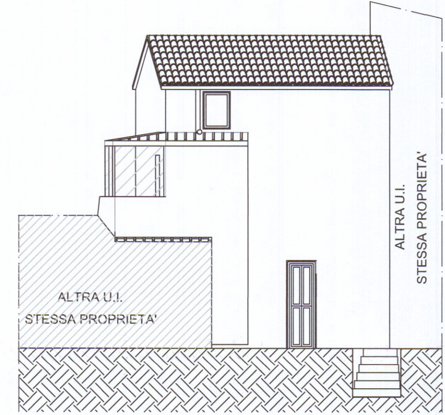
PROSPETTO SUD OVEST
