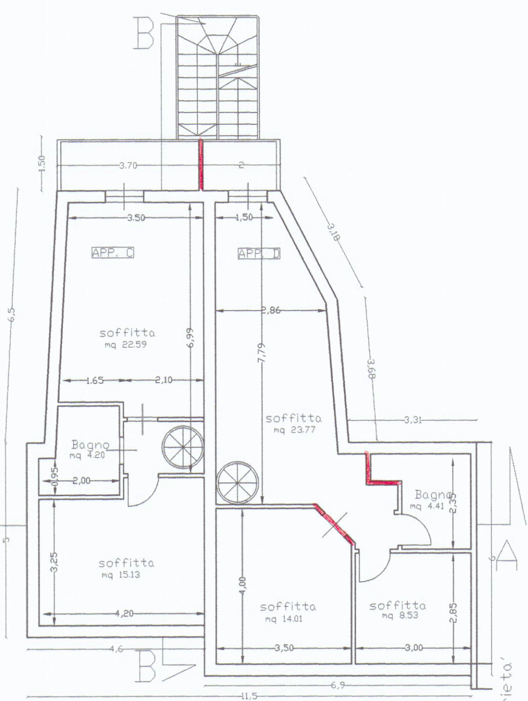
PIANO SOTTOTETTO
