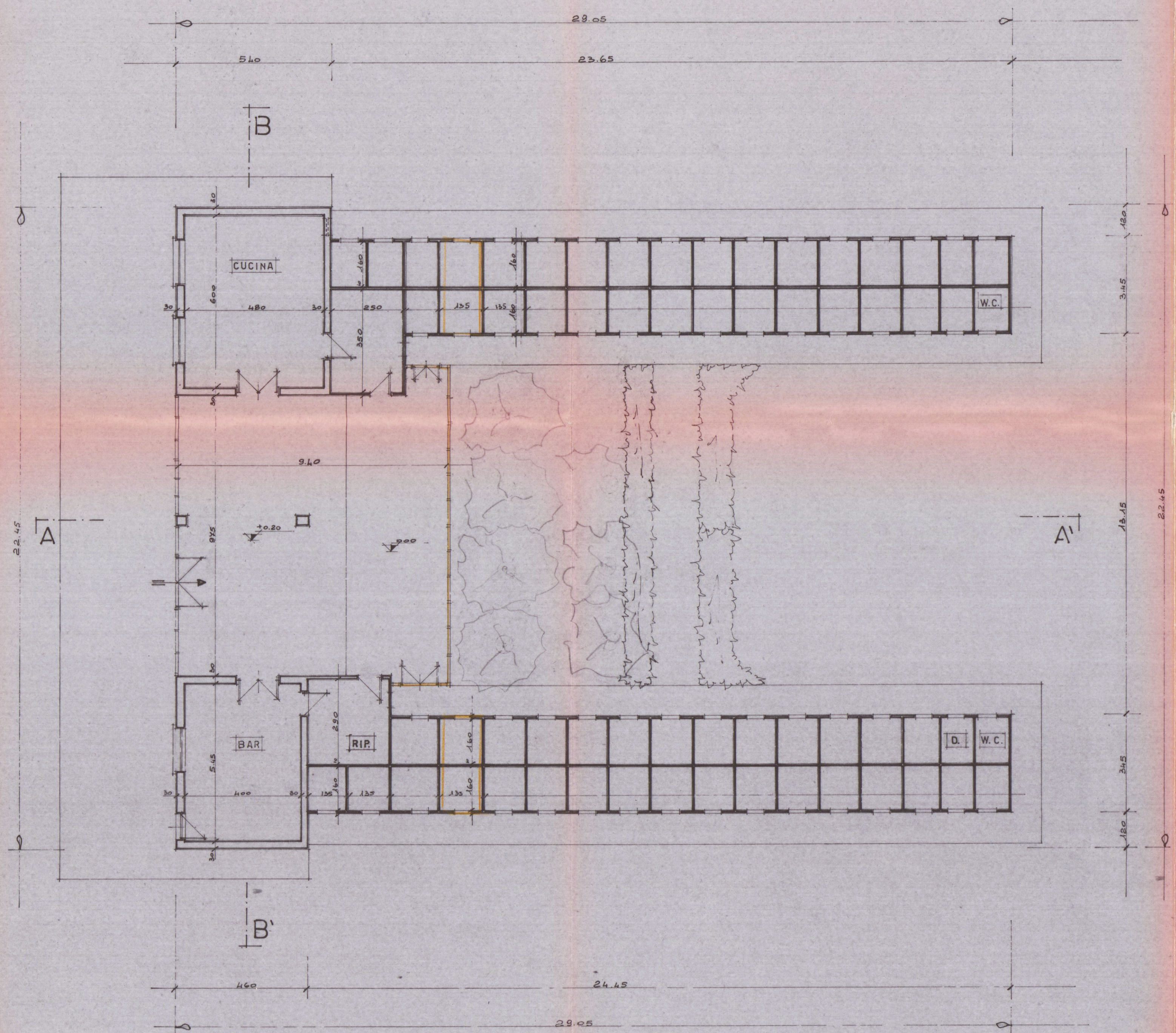
Pianta
