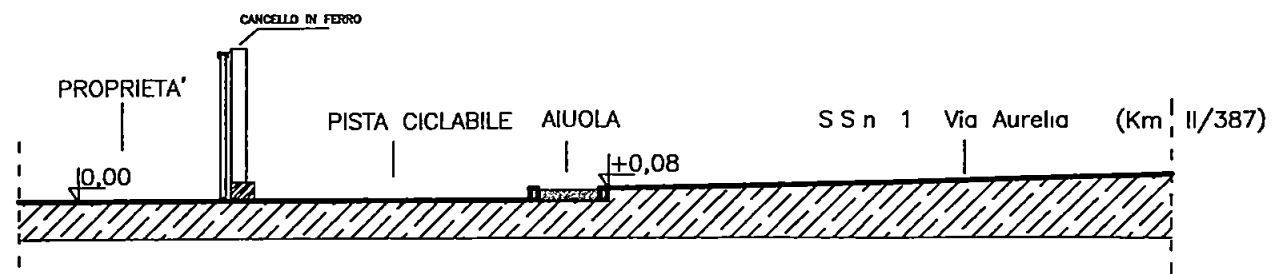
SEZIONE A A
