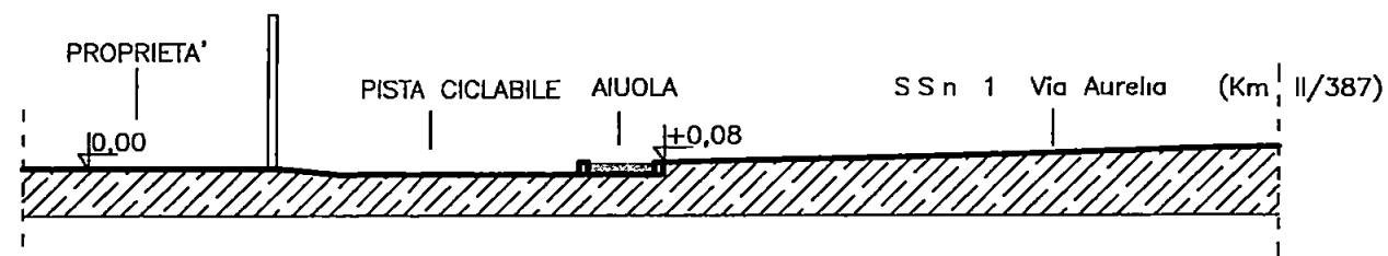
SEZIONE A A
