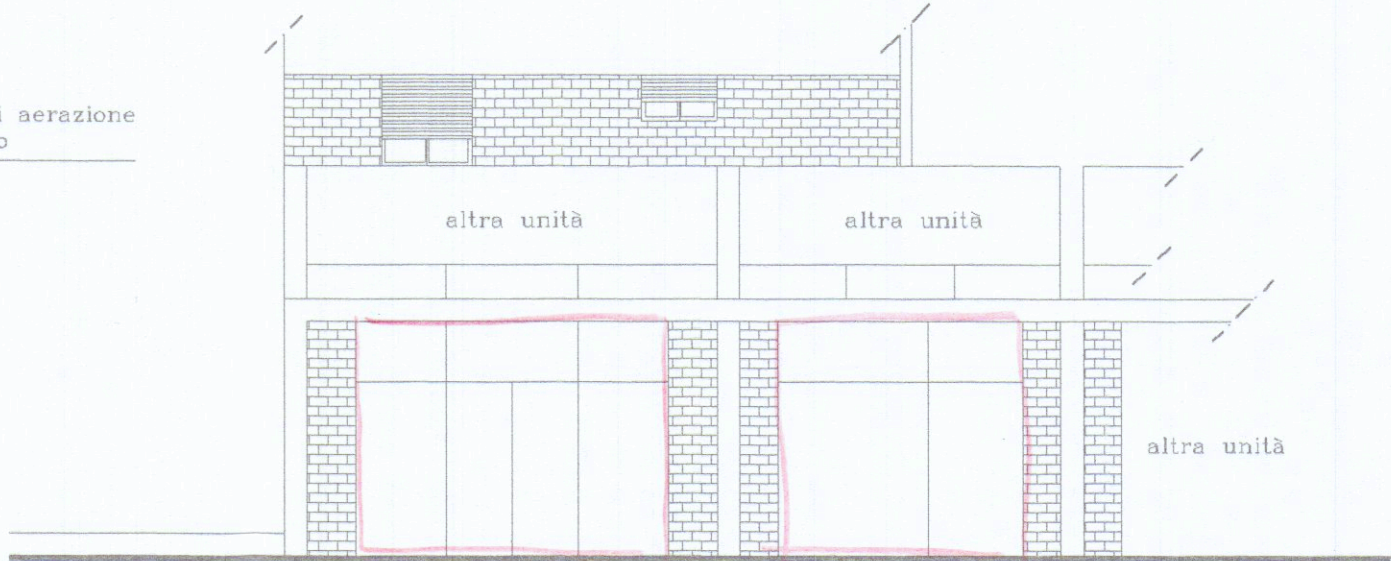
PROSPETTO LATO VIALE XX SETTEMBRE
