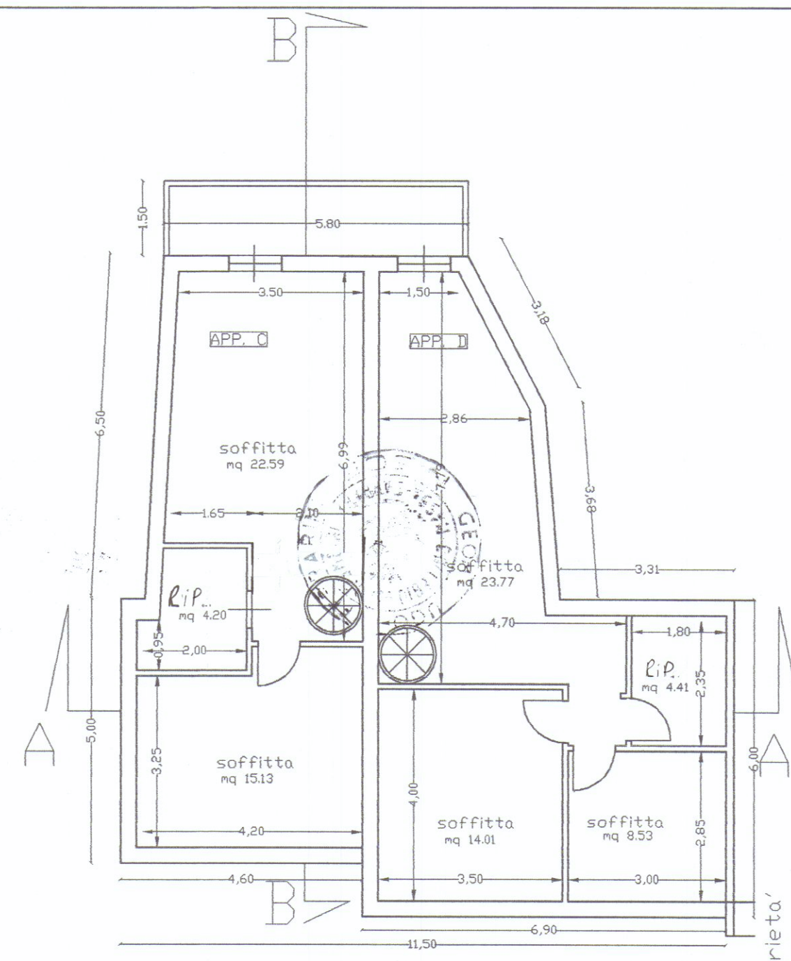
PIANO SOTTOTETTO
