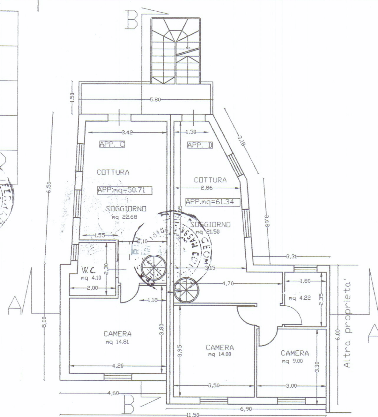
PIANO PRIMO
