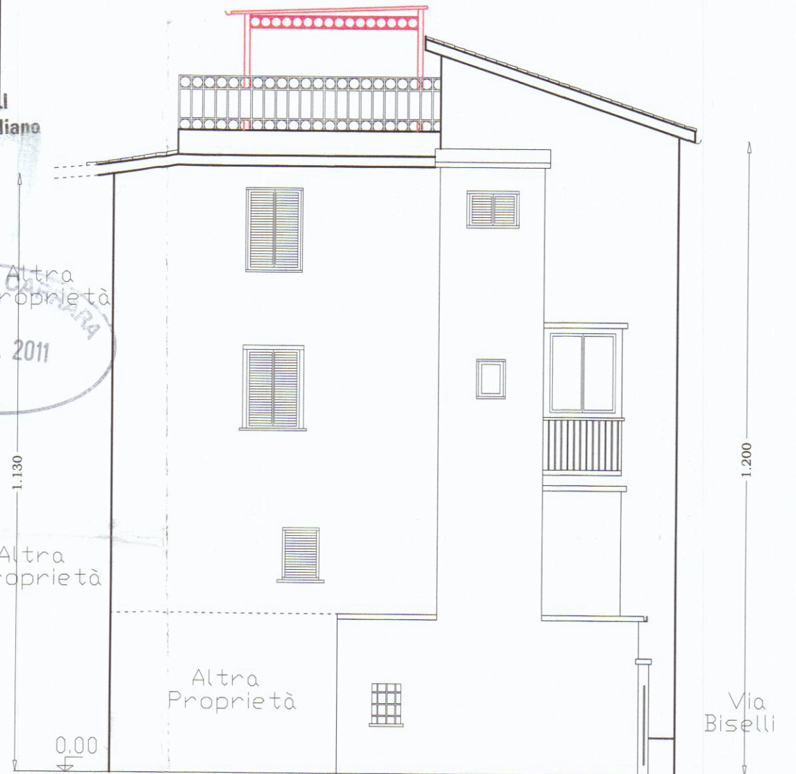
PROSPETTO NORD - OVEST
