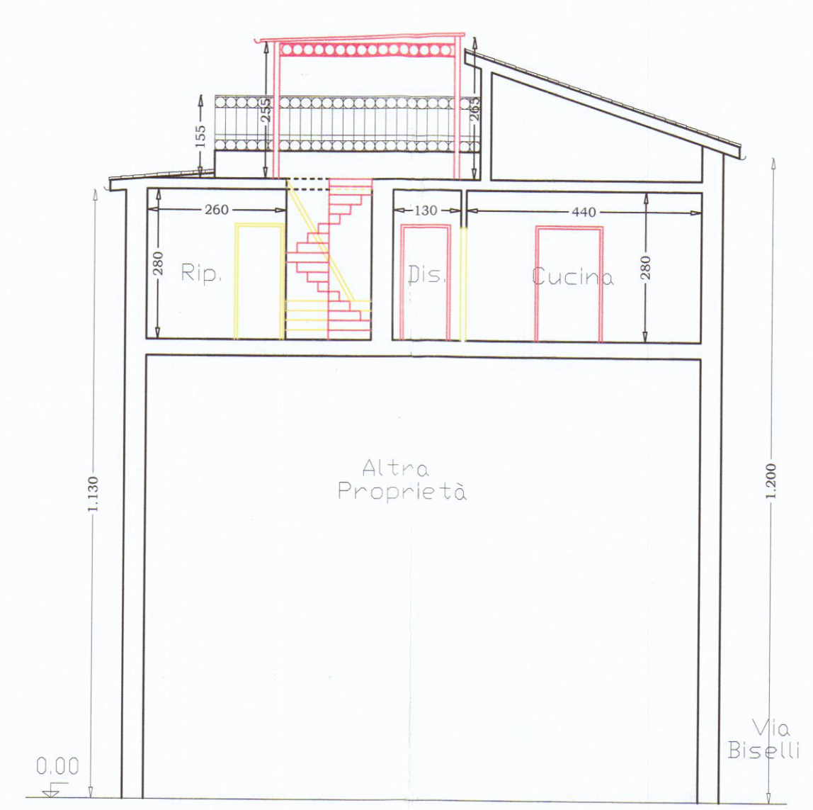
Sezione A-A'
