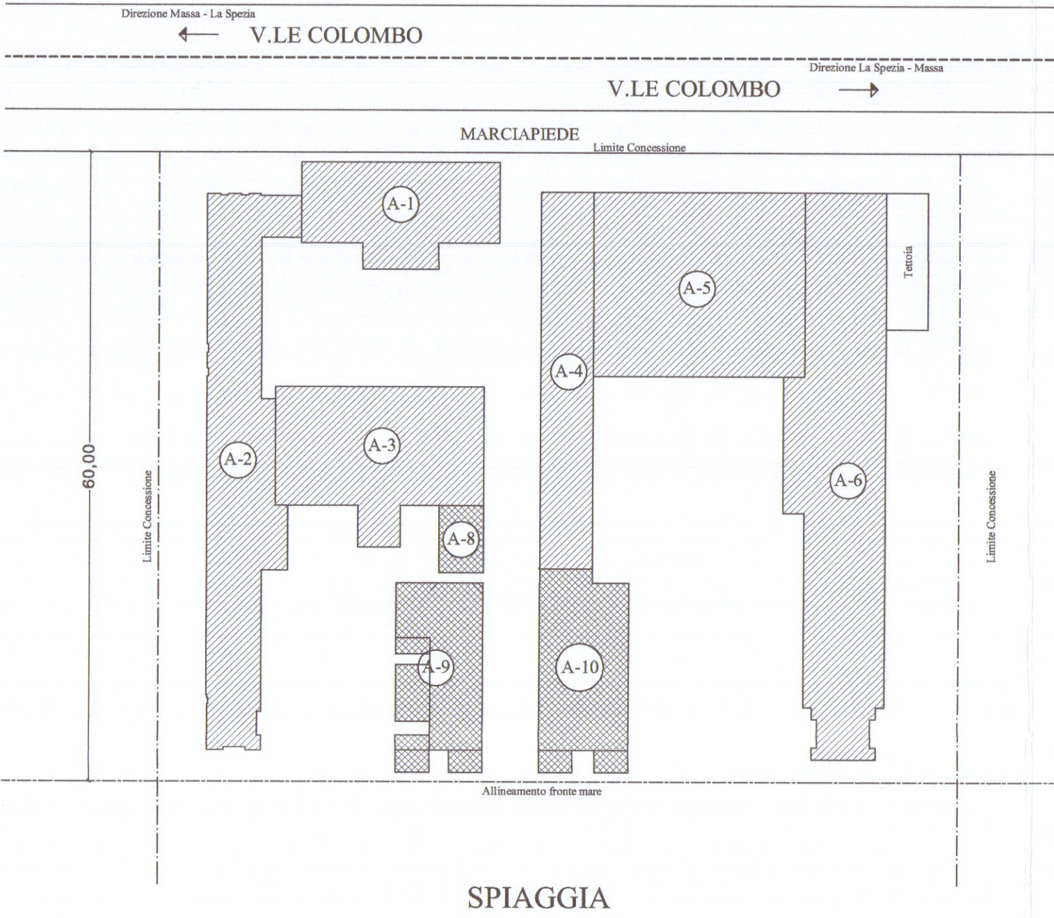
PLANIMETRIA GENERALE SCALA 1 : 500
