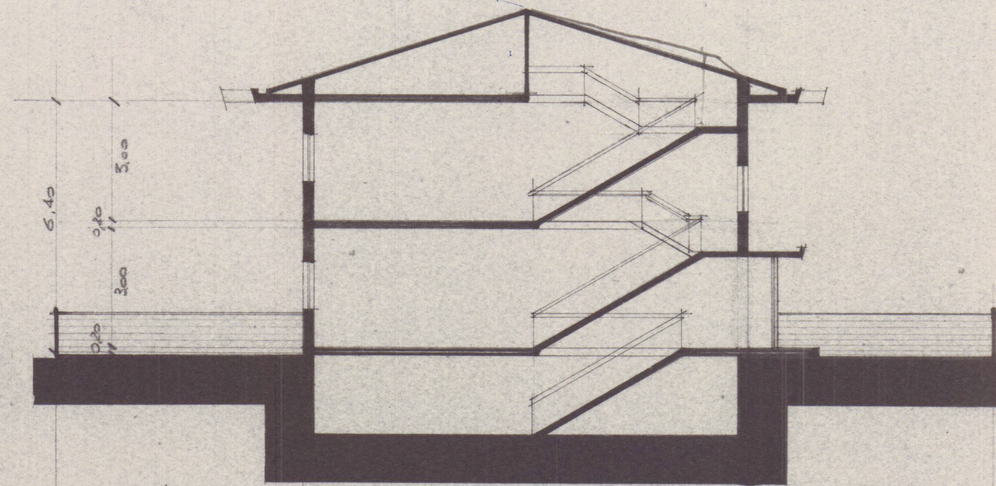
SEZ. A-B
