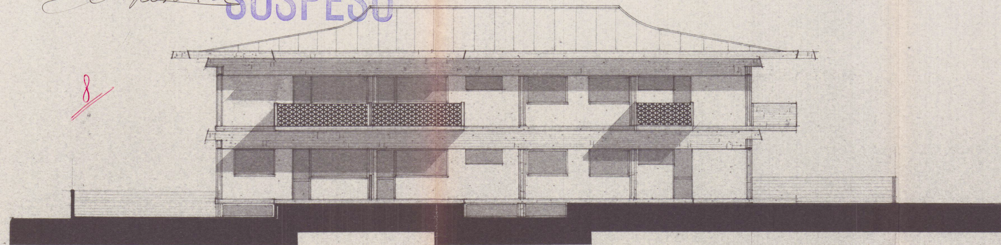
PROSPETTO OVEST 6,40
