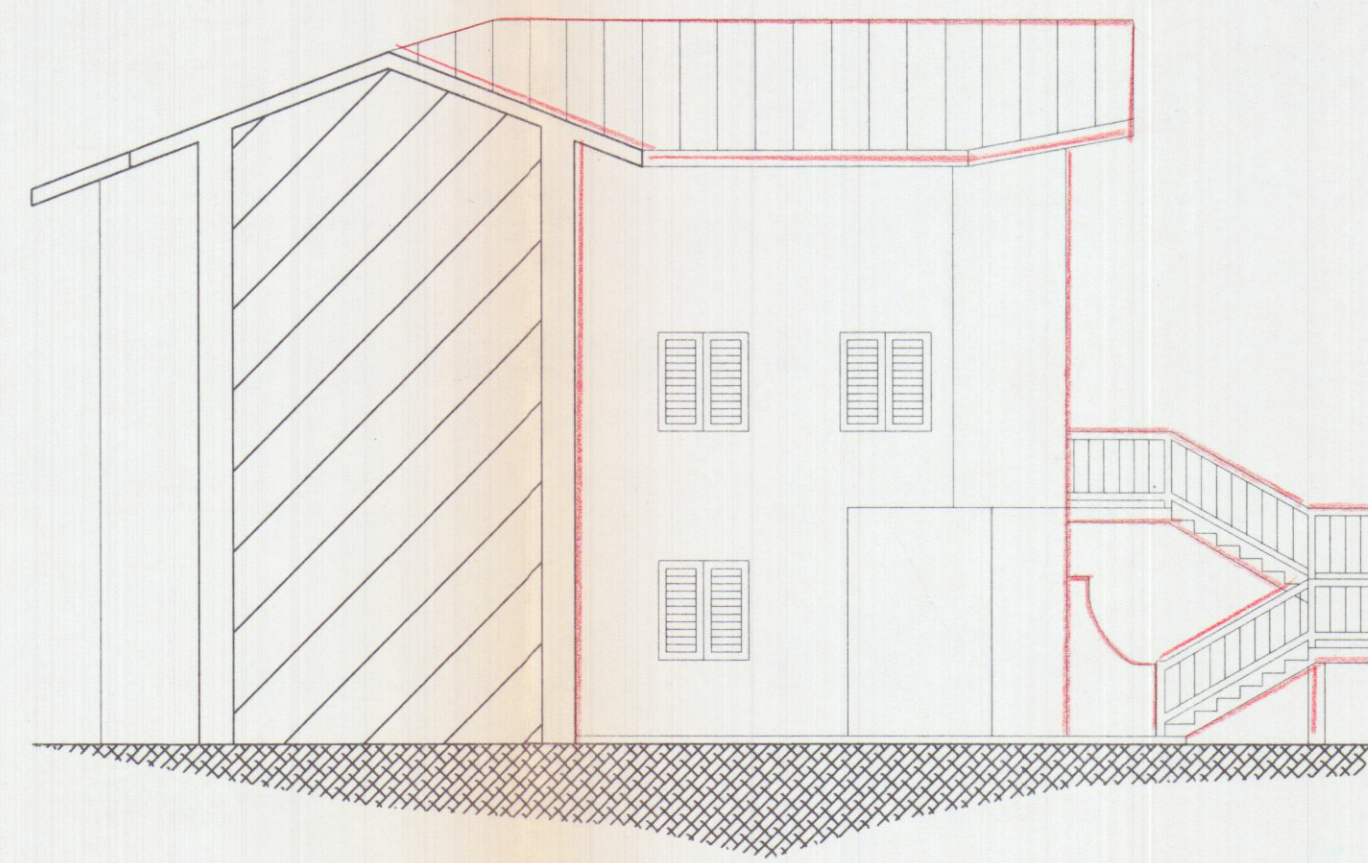
PROSPETTO OVEST
