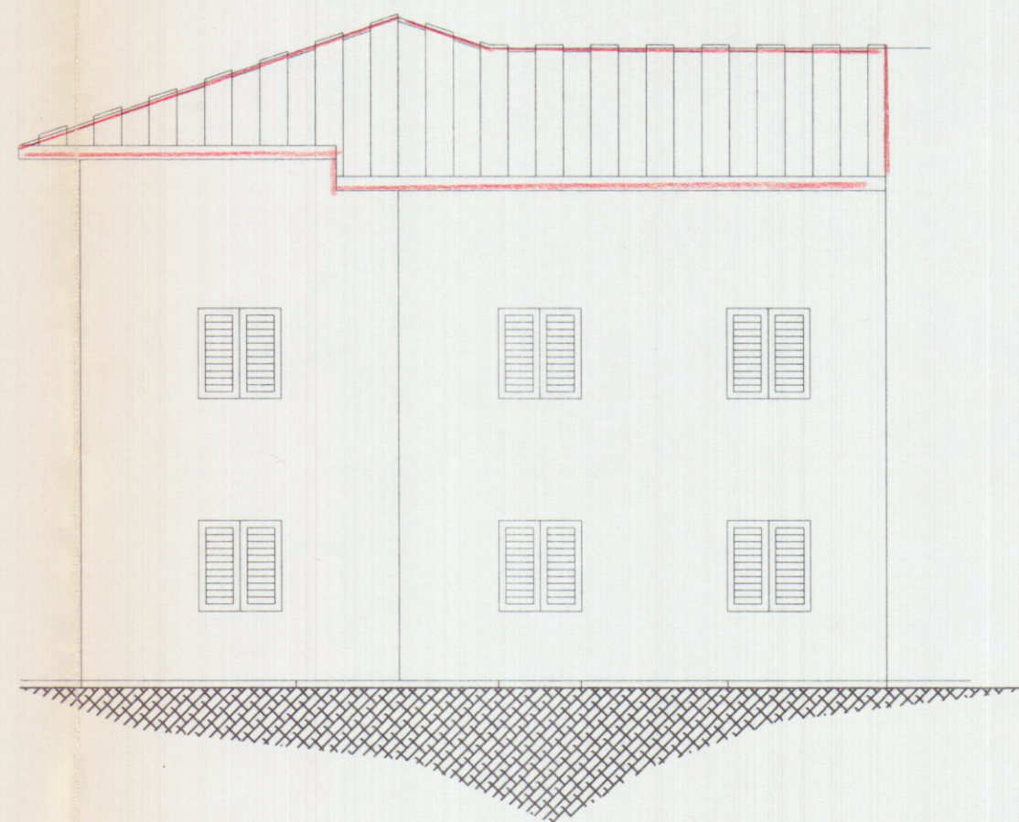
PROSPETTO NORD
