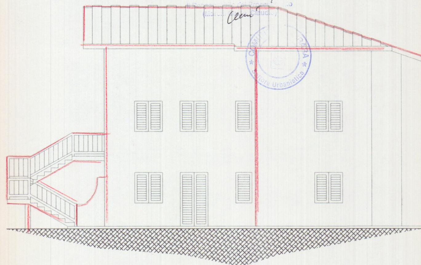
PROSPETTO EST
