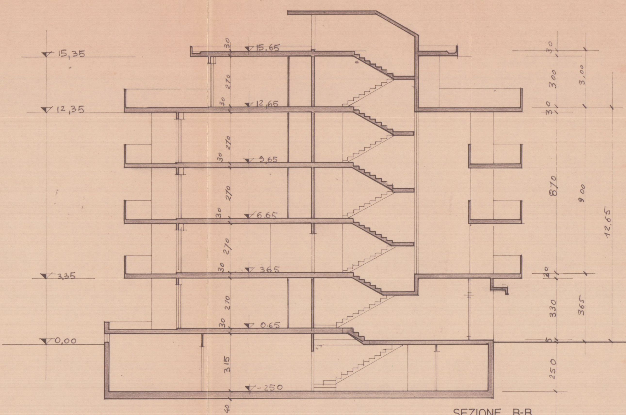
SEZIONE B-B
