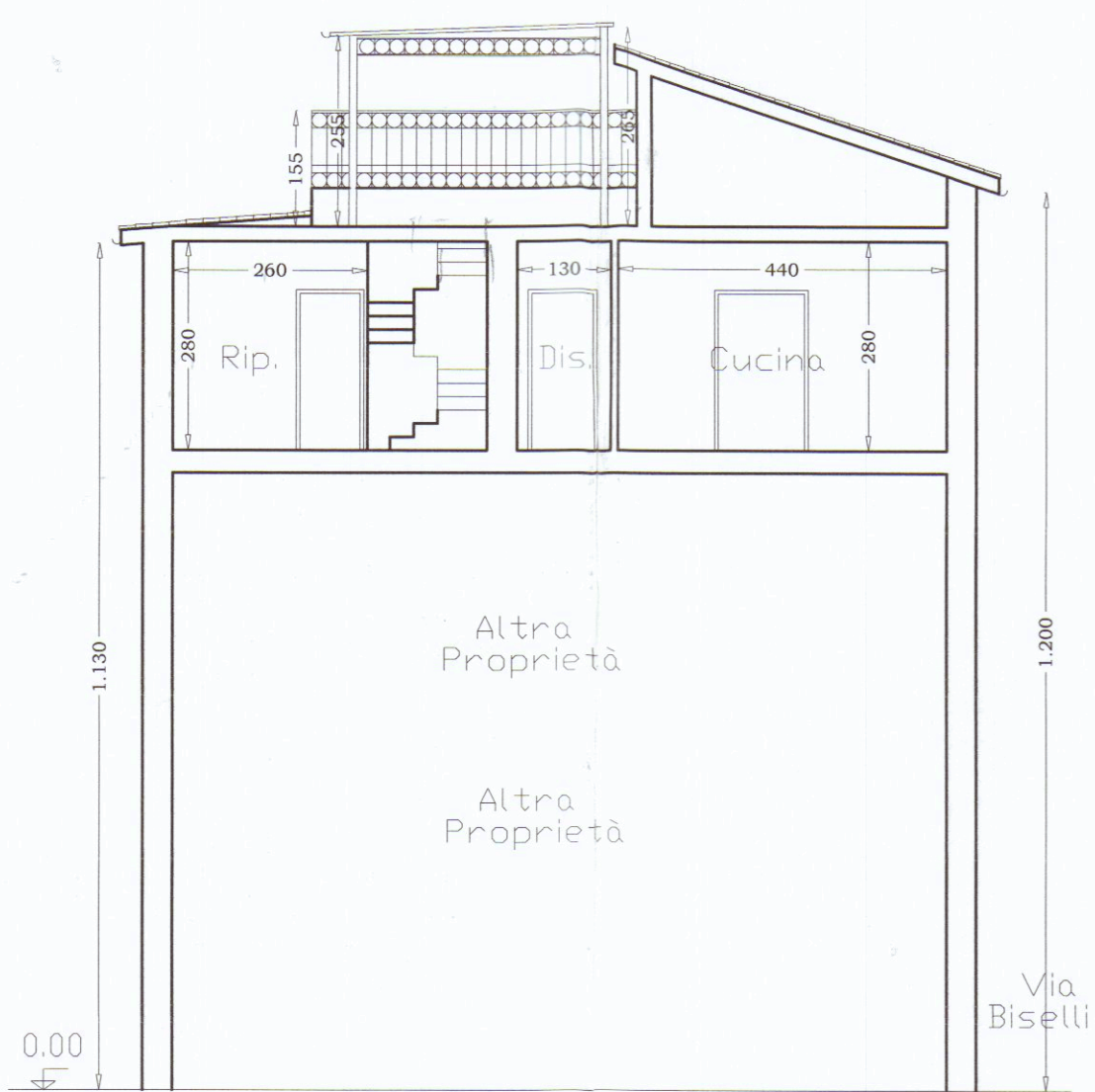
Sezione A-A'
