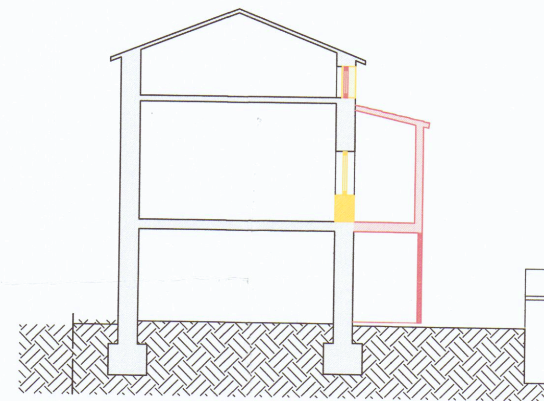
SEZIONE A-A
