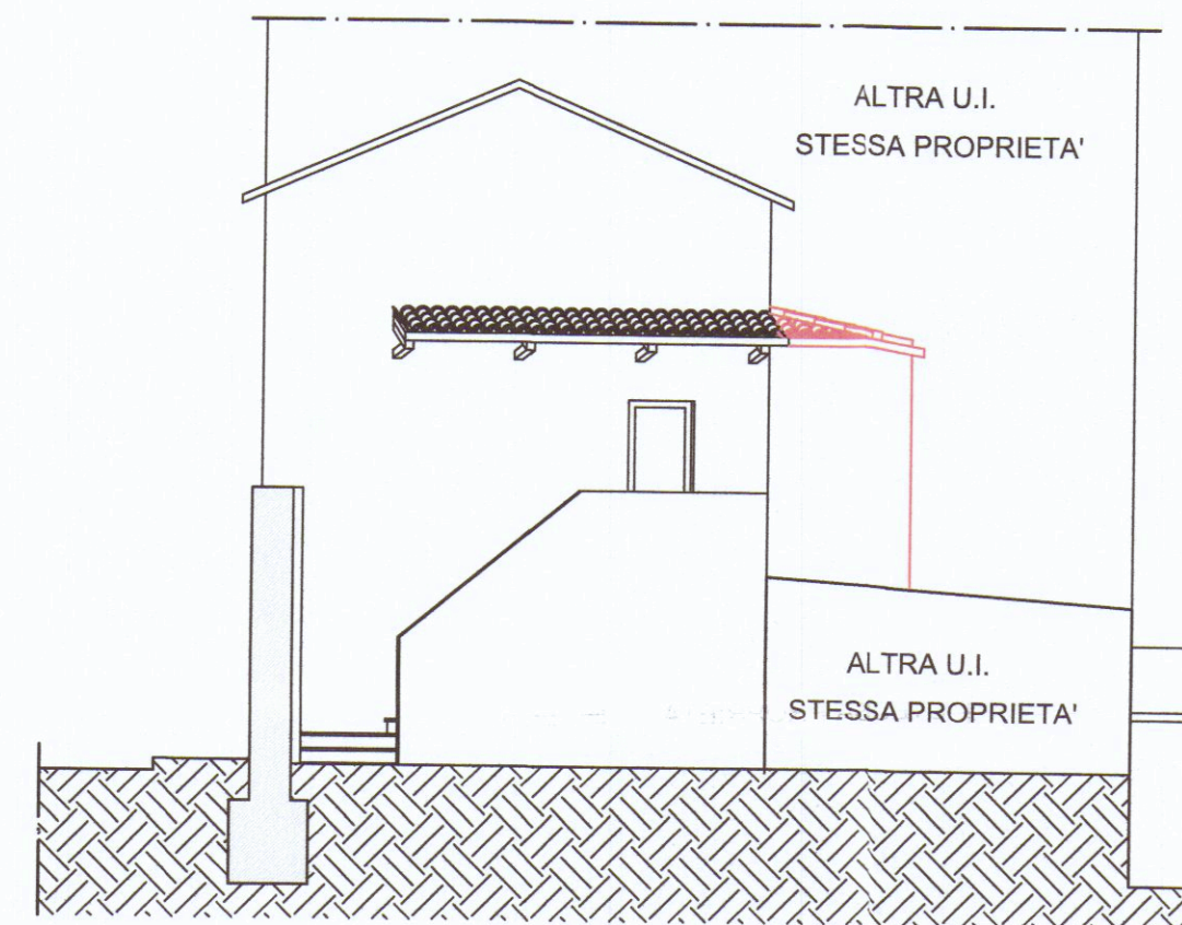
PROSPETTO OVEST
