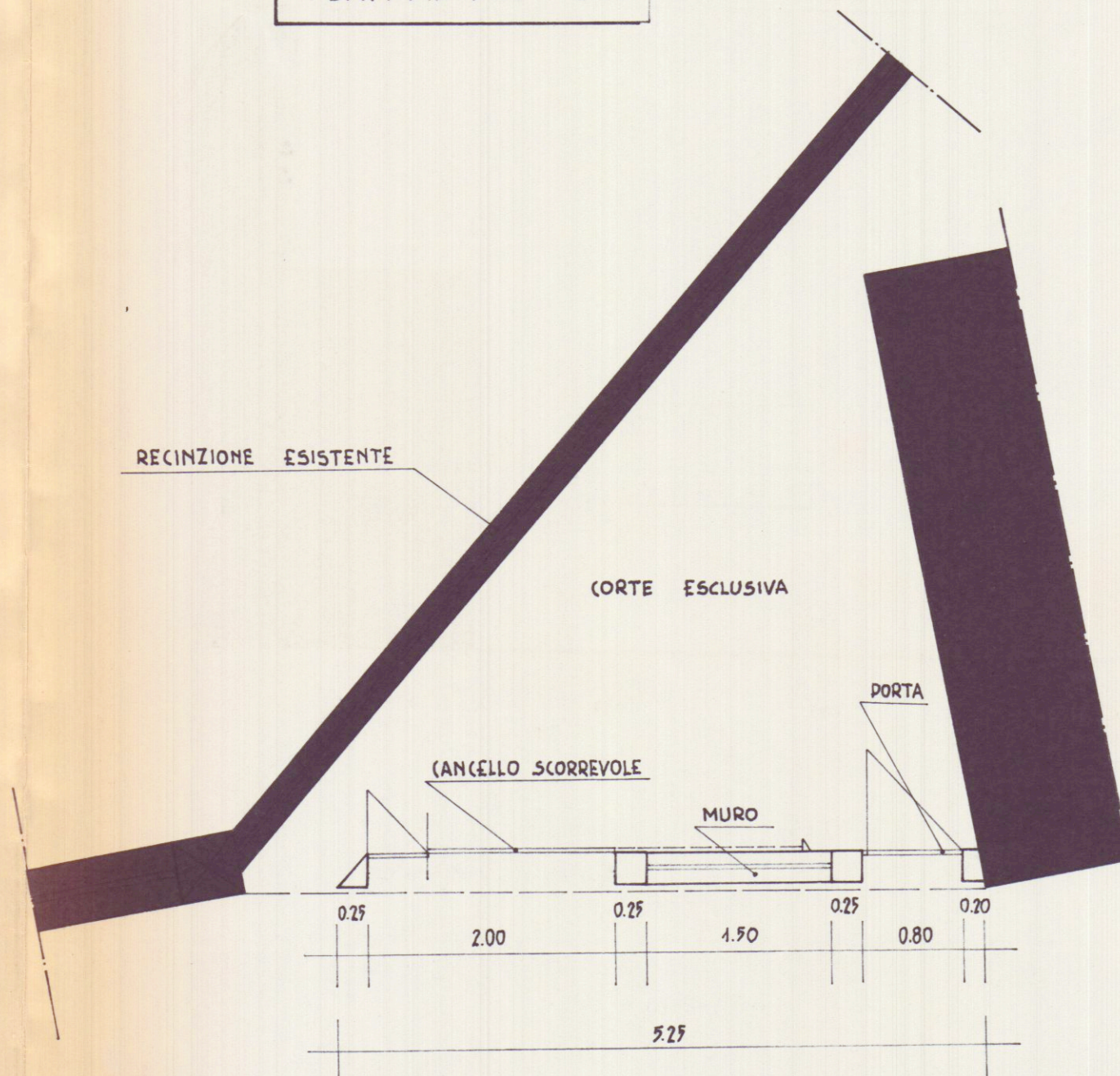
PLANIMETRIA 1:50
