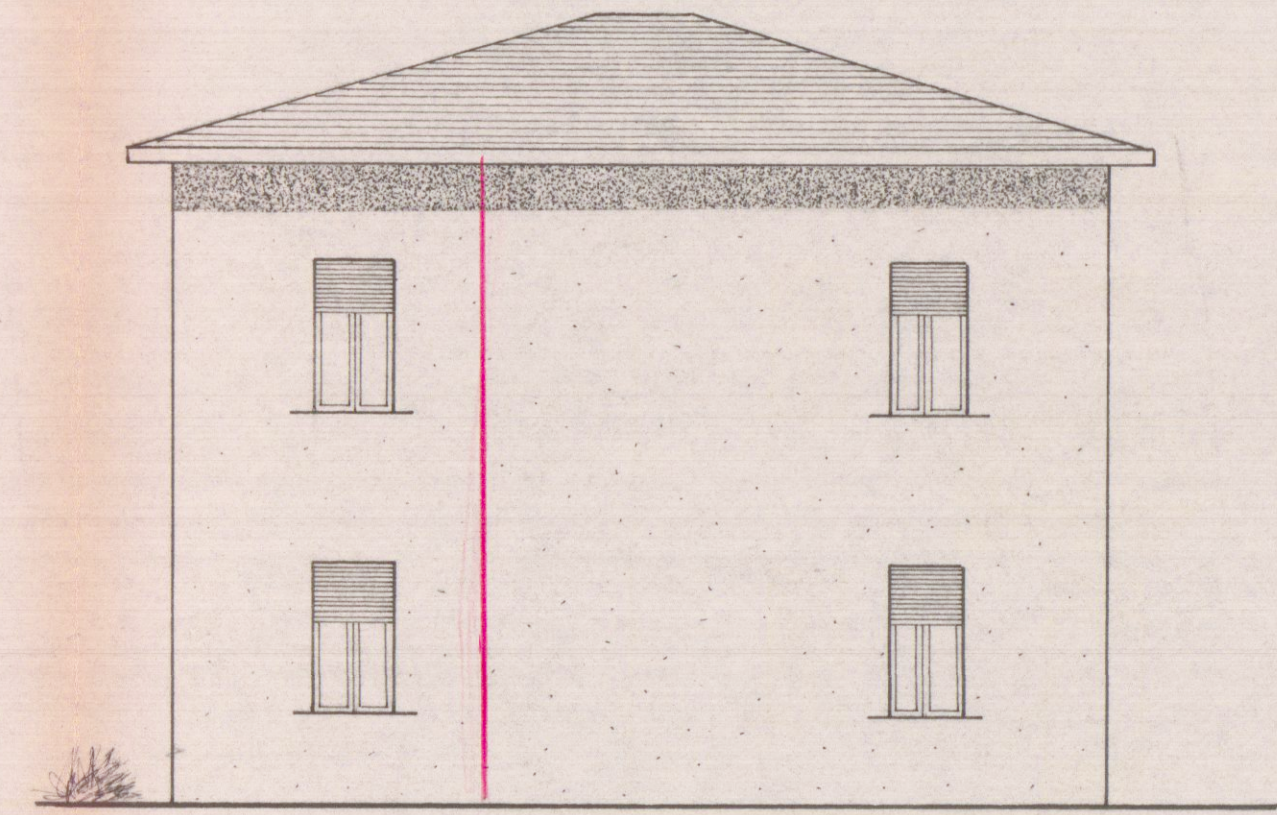
PROSPETTO OVEST
