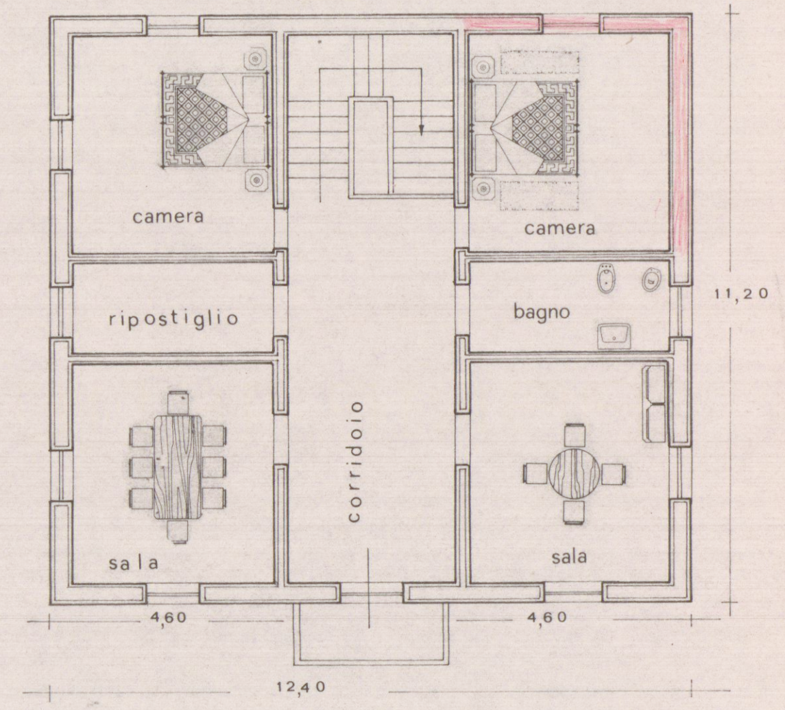
PIANTA 1° PIANO
