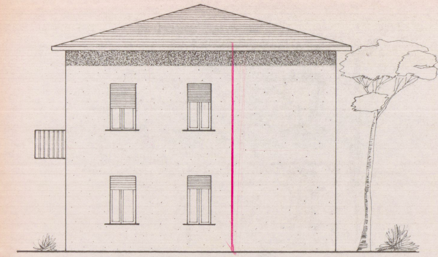
PROSPETTO NORD
