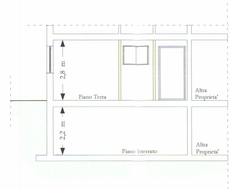
SEZIONE A-A
