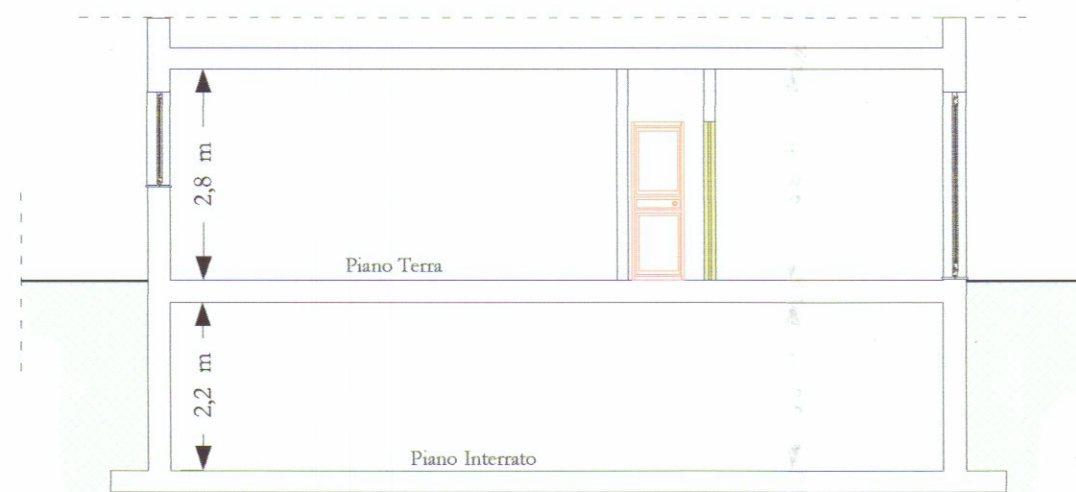
SEZIONE B-B Raffronto
