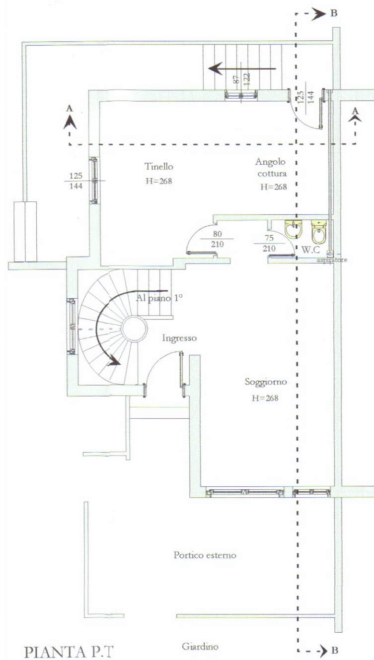
PIANTA P.T
