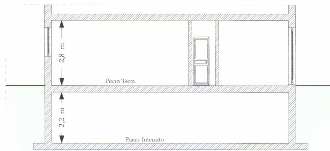
SEZIONE B-B Progetto
