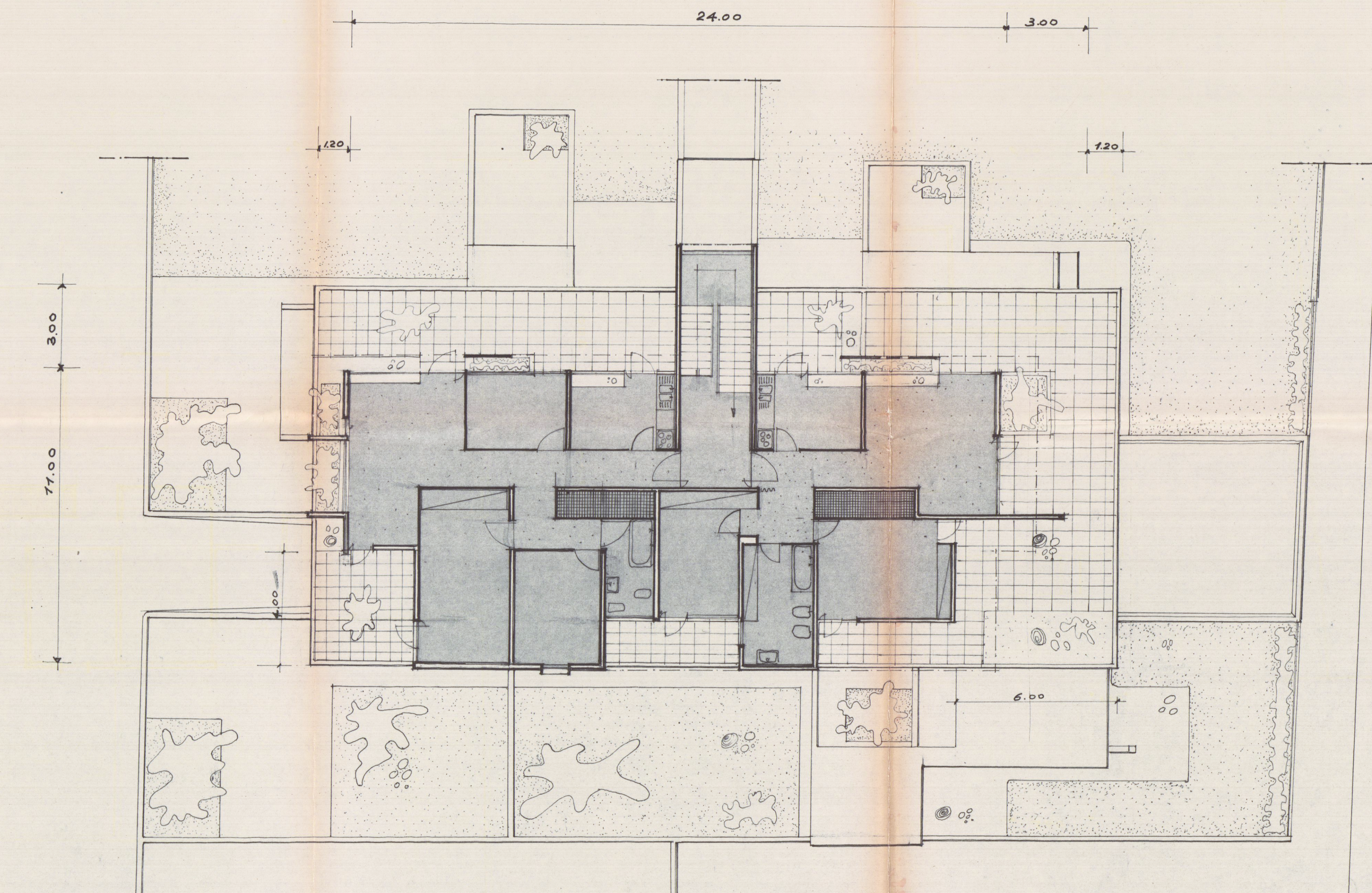
PIANTA PIANO ATTICO SUP. COPERTA mq. 233 + TERRAZZI mq. 175
