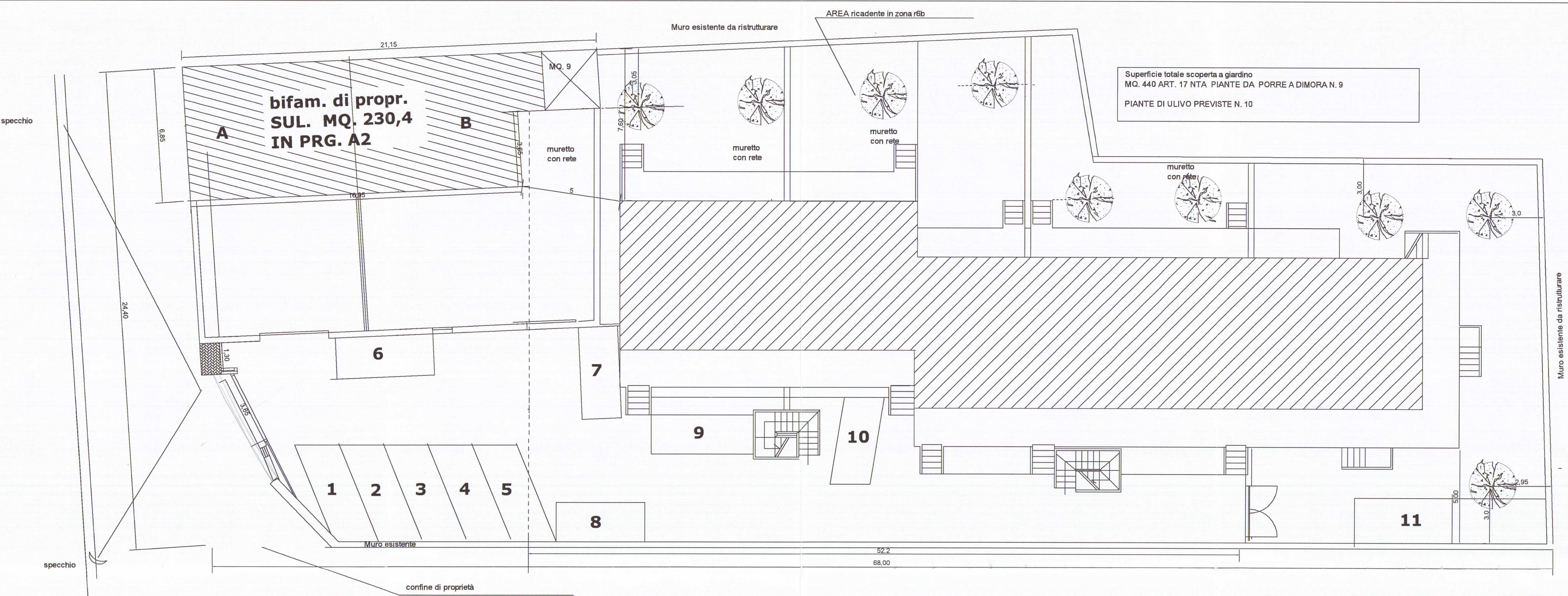
PLANIMETRIA GENERALE SCALA 1:100
