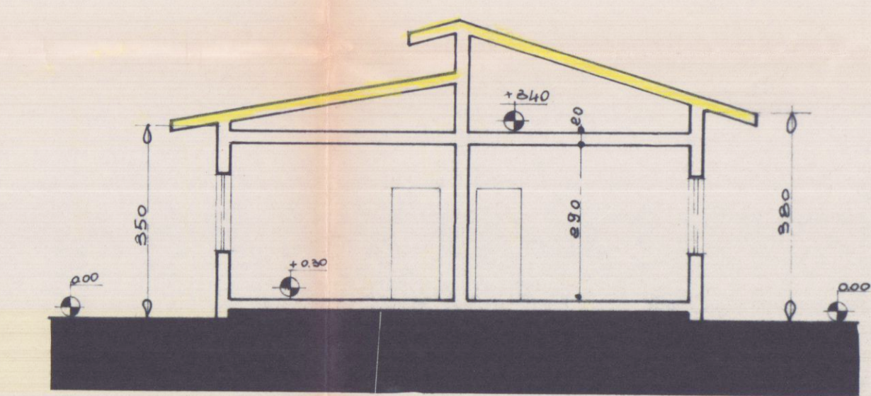
SEZIONE A-A
