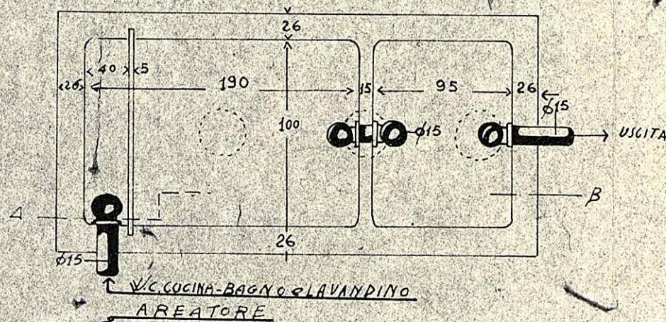
PIANTA
