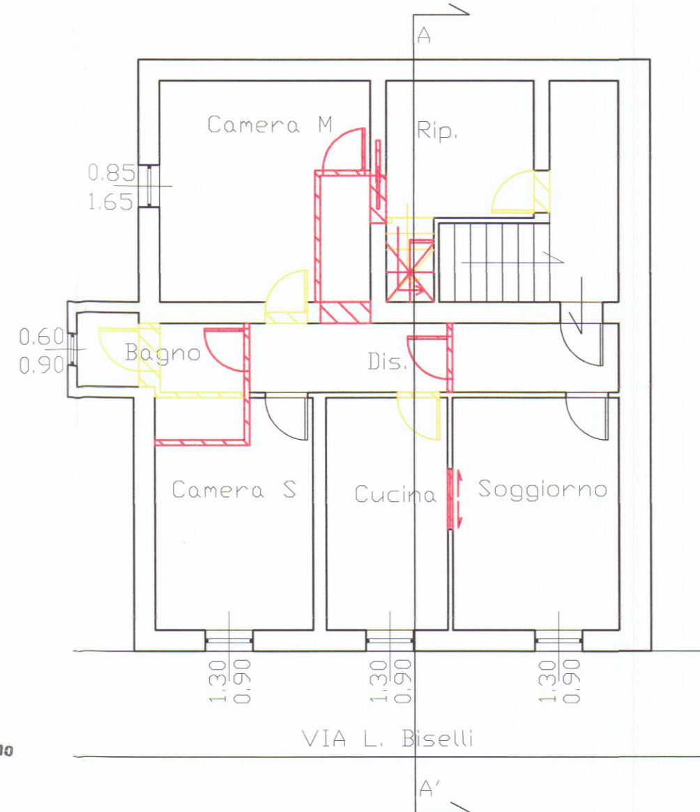
Pianta Piano Terzo
