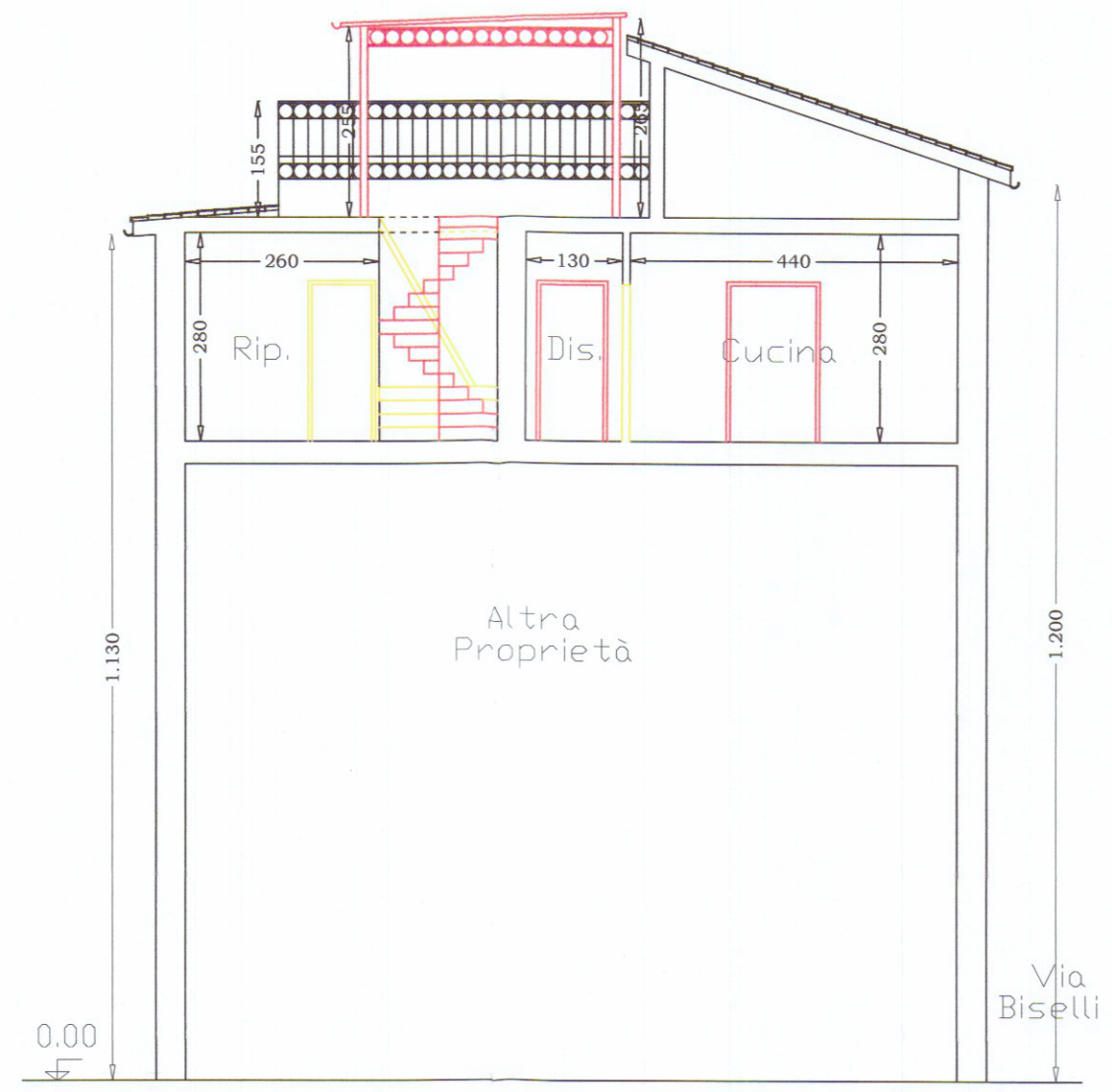
Sezione A-A'
