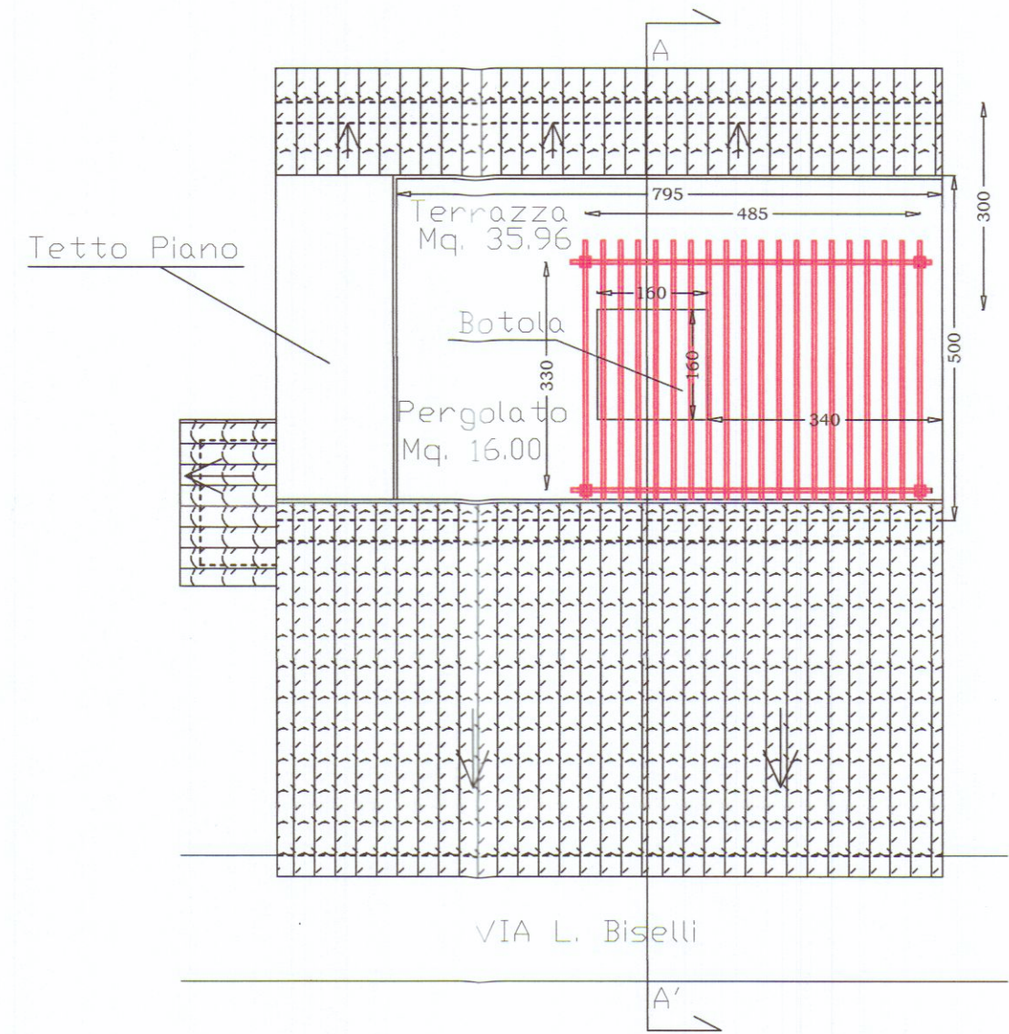
Pianta Copertura
