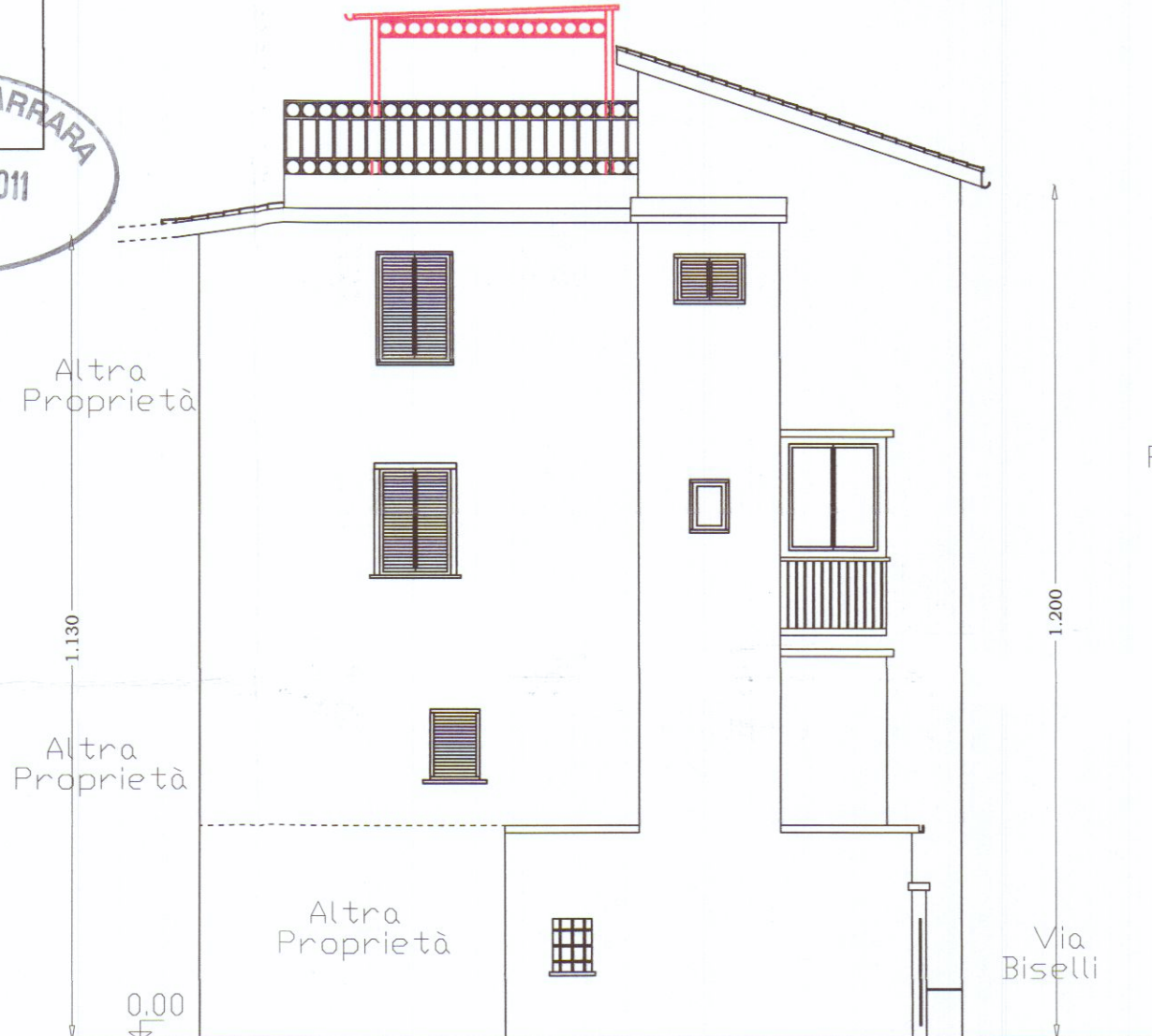
PROSPETTO NORD - OVEST
