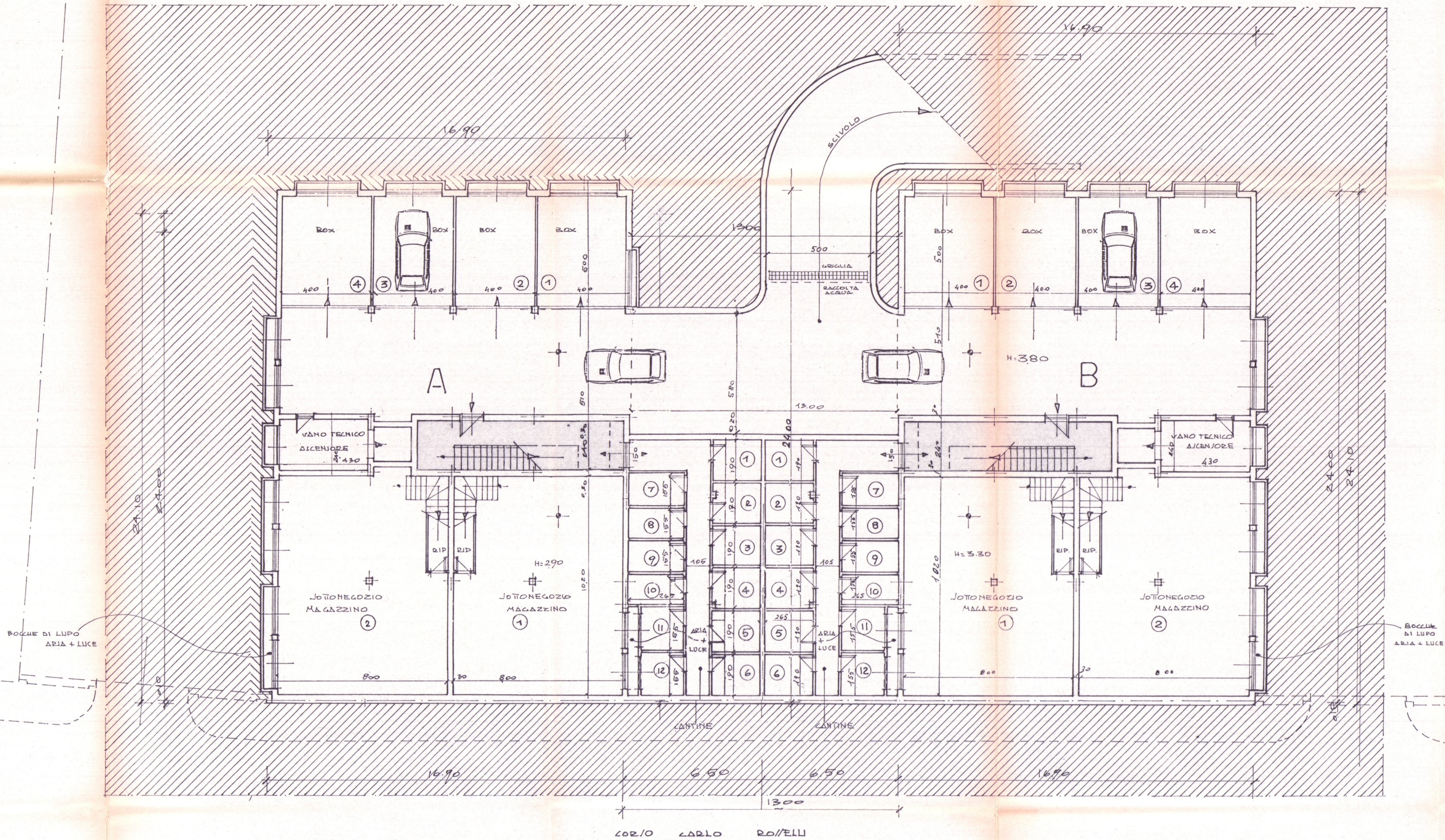
PIANTA PIANO SCANTINATO
