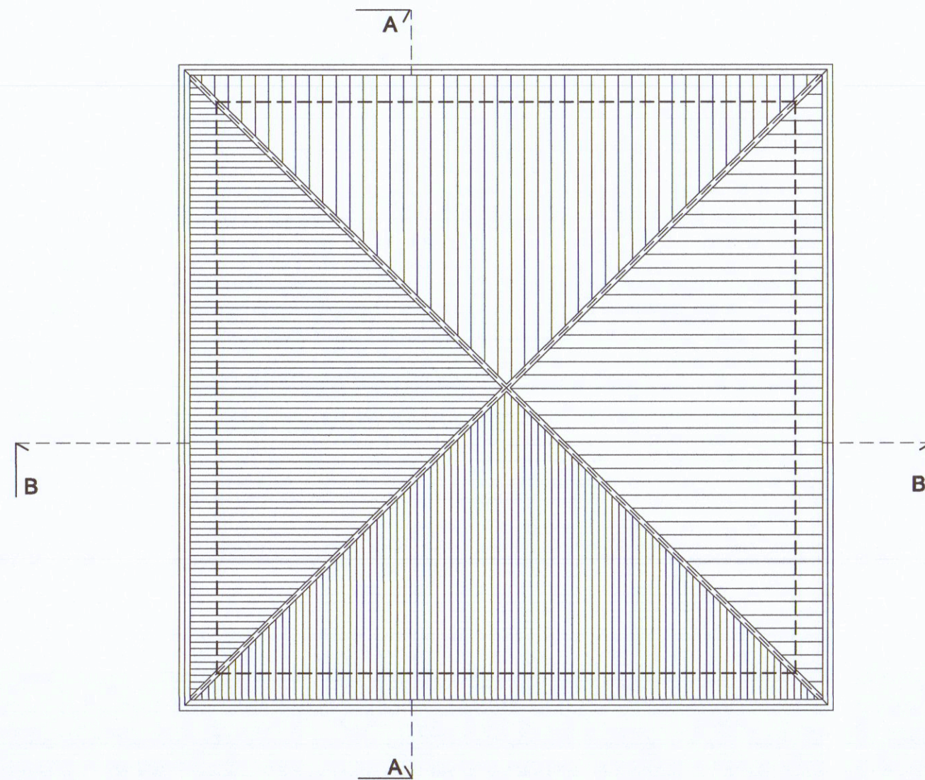
PIANTA COPERTURA
