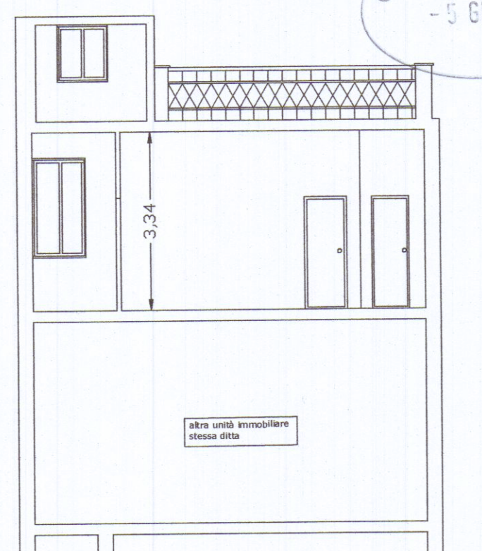
SEZIONE B-B
