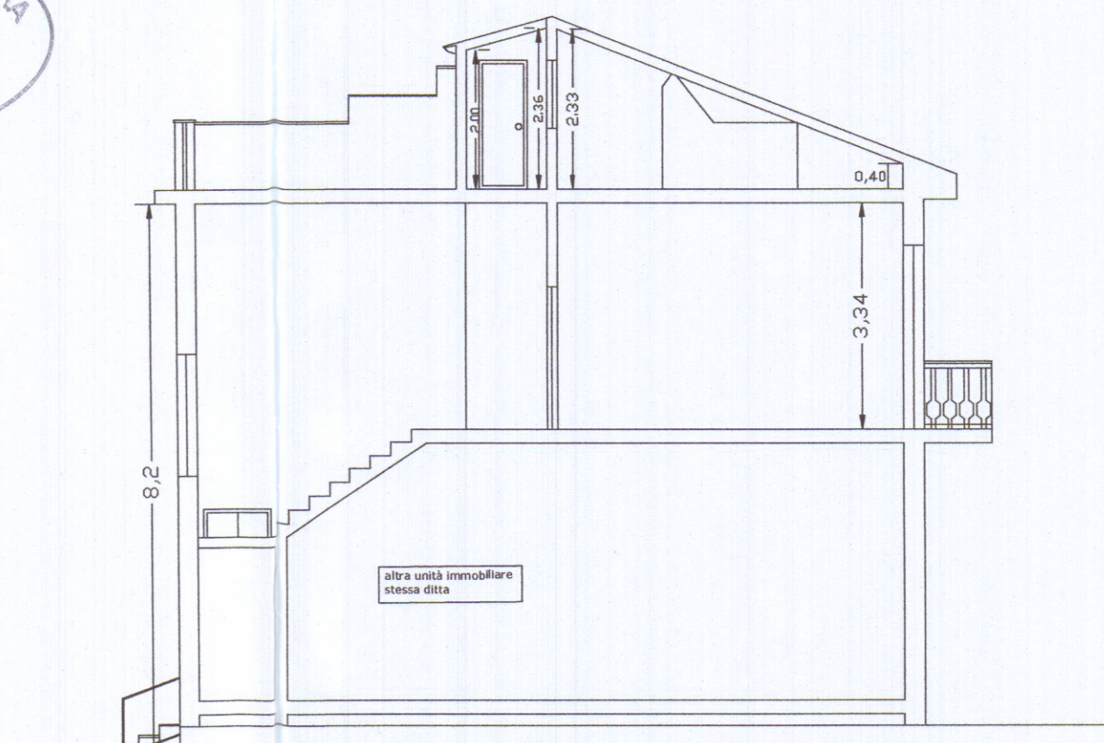
SEZIONE A-A
