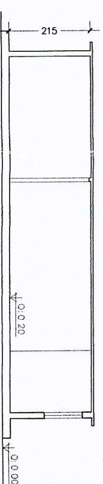
Sezione B-B
