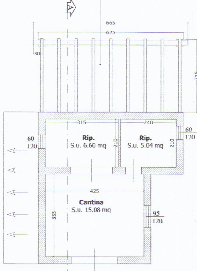
PIANO TERRA CASETTA
