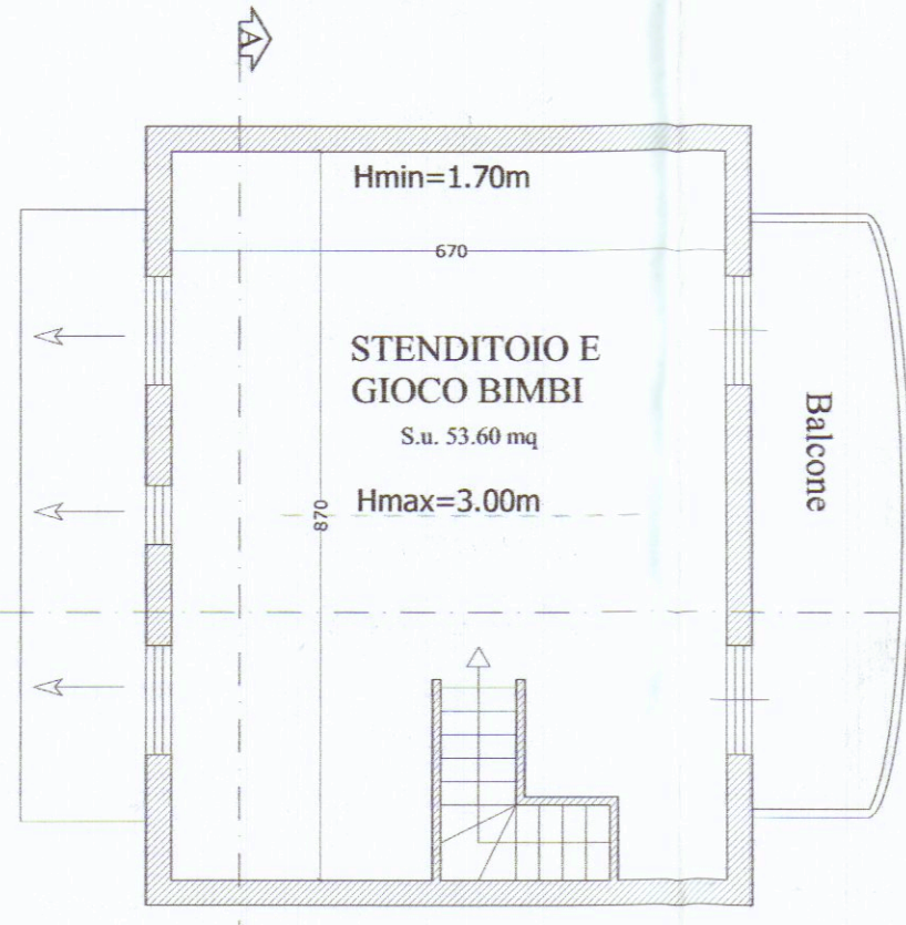
PIANO PRIMO
