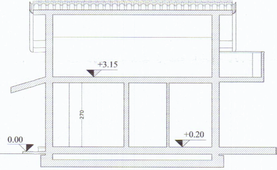
SEZIONE B-B
