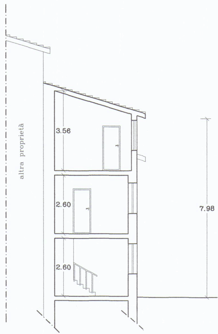
SEZIONE A - A
