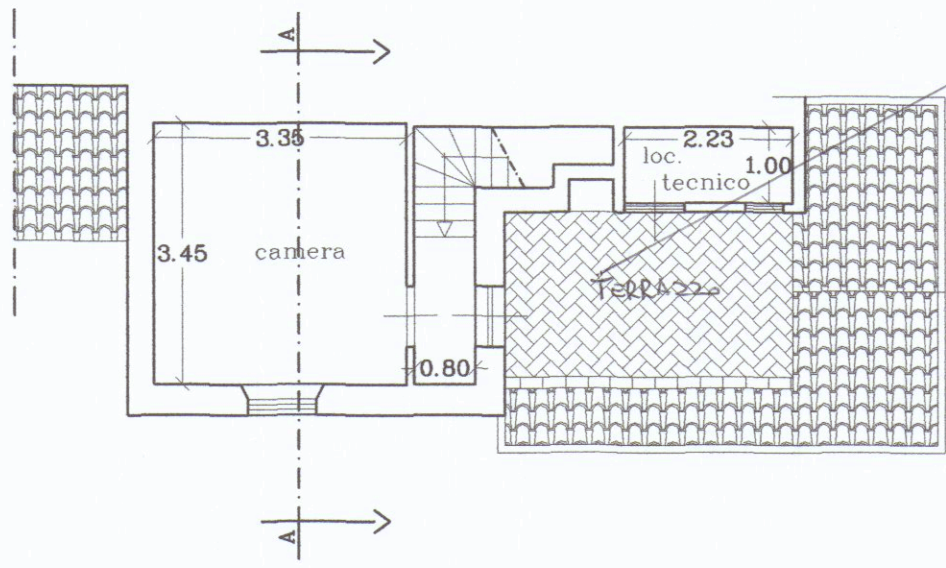
PIANO SECONDO
