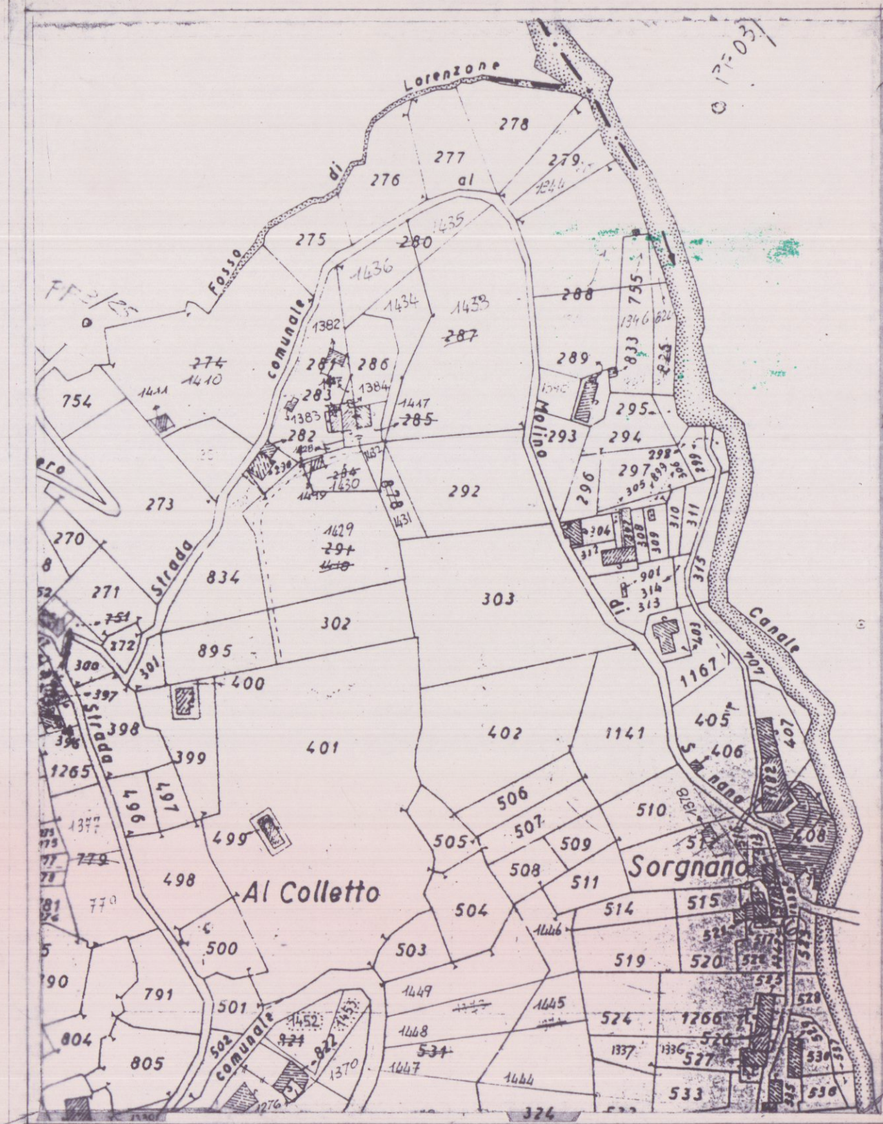
STRALCIO PLANIMETRICO CATASTALE FOGLIO 30 SCALA 1:2000 MAPP. 206, 1417, 501b, 1-2, 1436, 1434, 1384, 1430, 1419, 1427, 1428, 1432 MAPP. 201, 203, 1382, 1383
