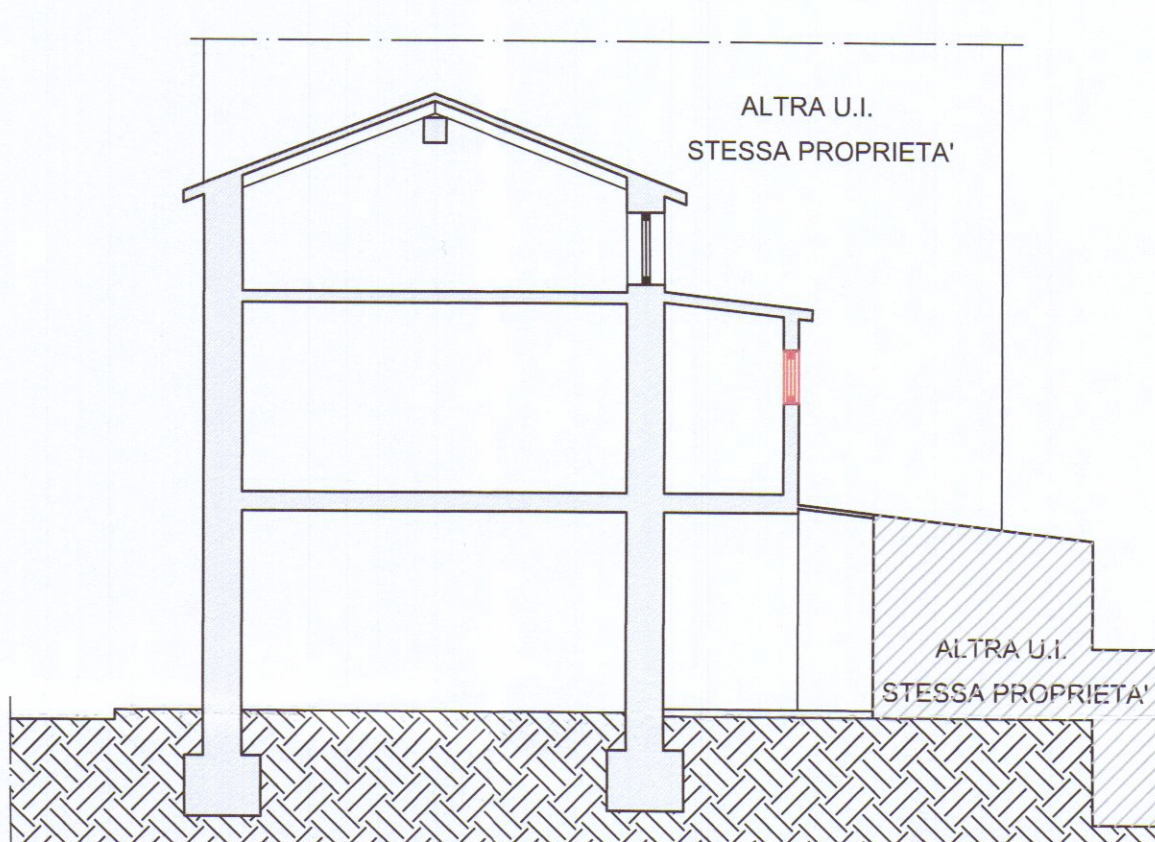
SEZIONE A-A
