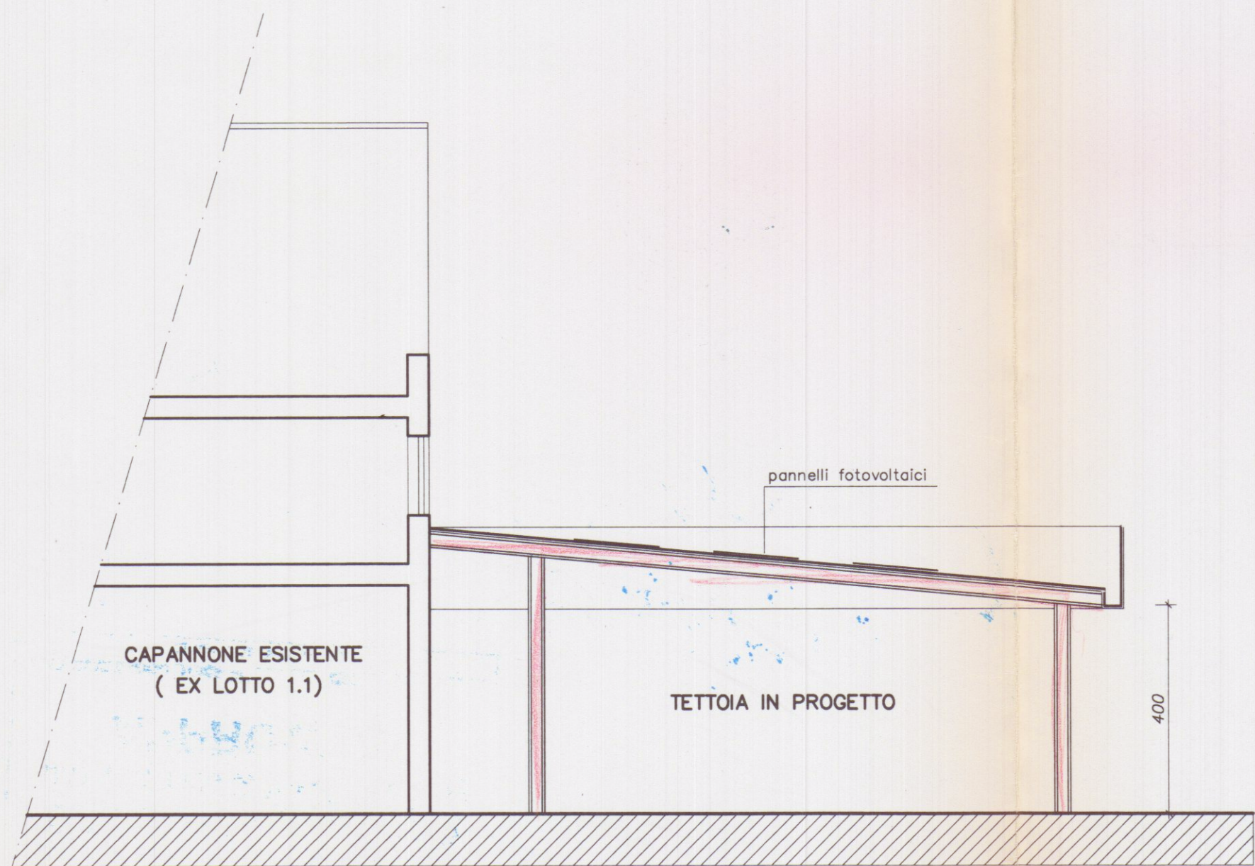
SEZIONE A A
