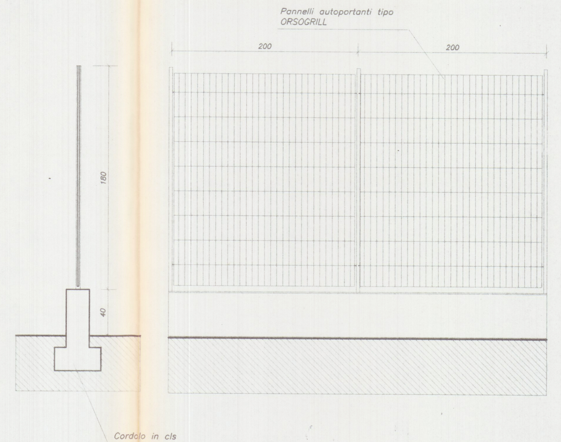
PARTICOLARE RECINZIONE scala 1/20
