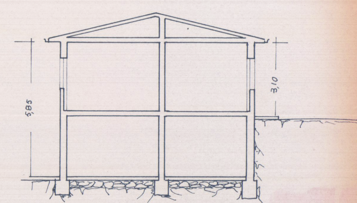
SEZIONE TRASVERSALE
