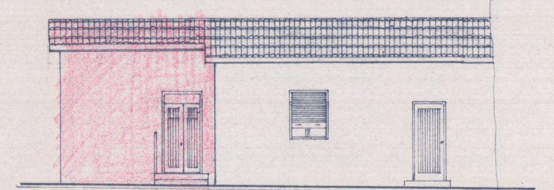
PROSPETTO NORD-EST
