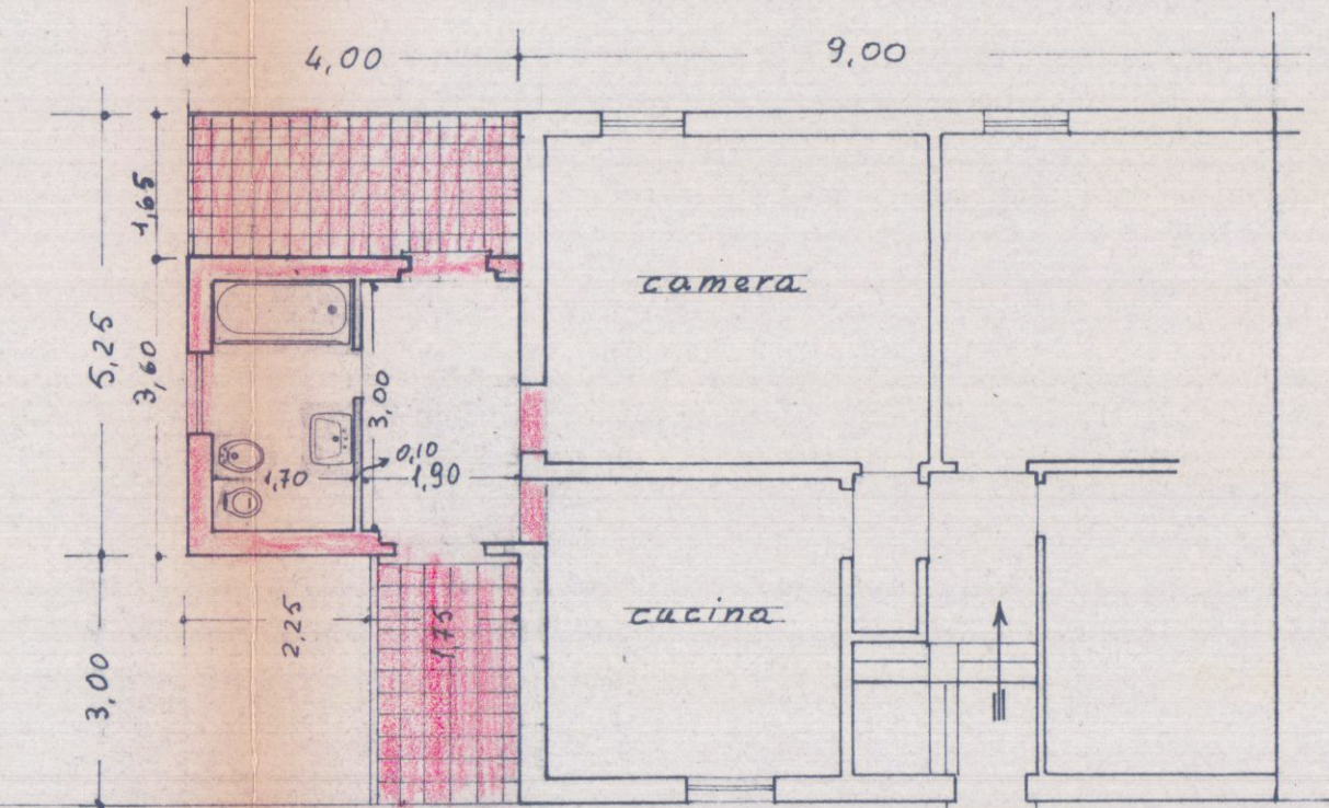
1° PIANO
