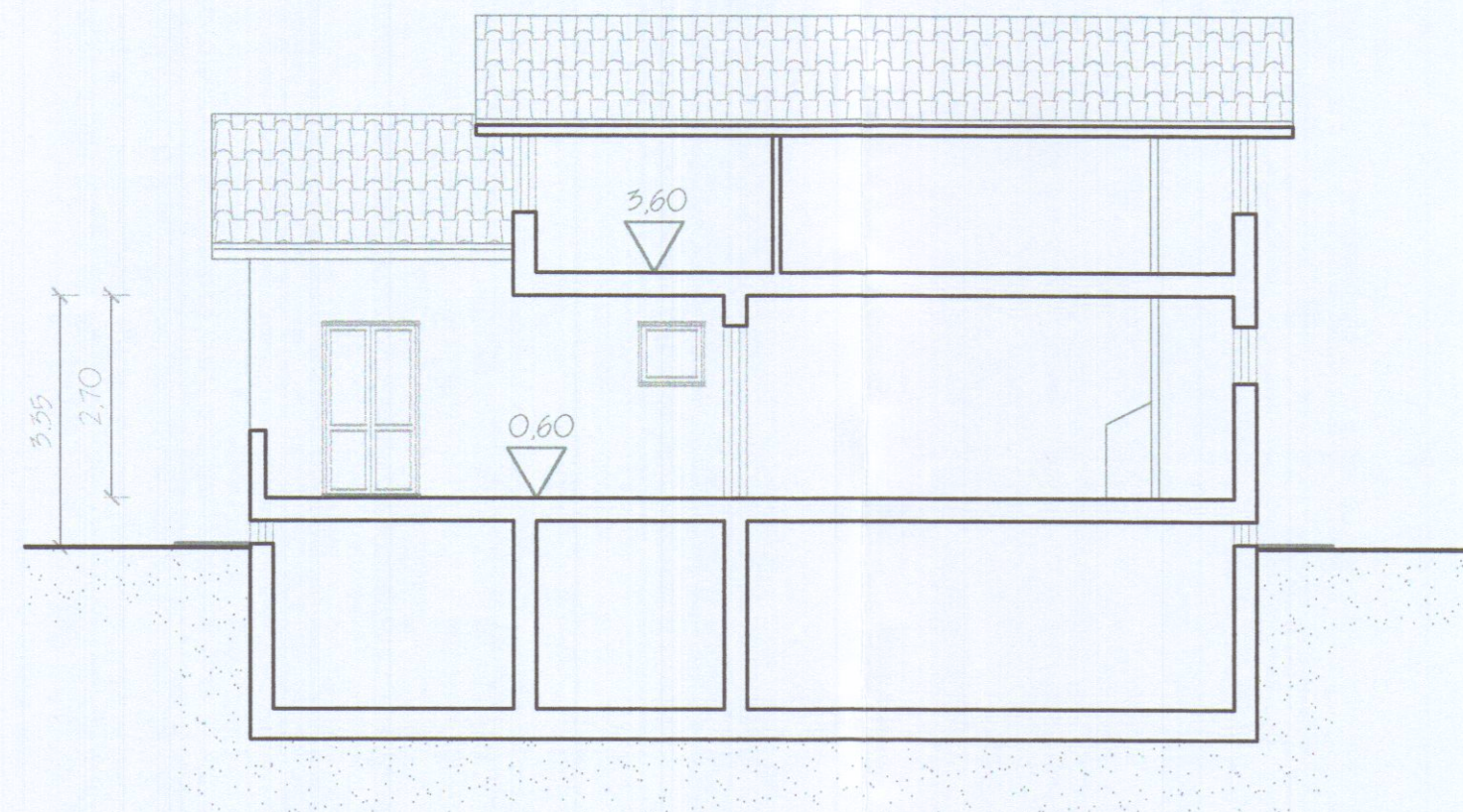
Sezione A-A'
