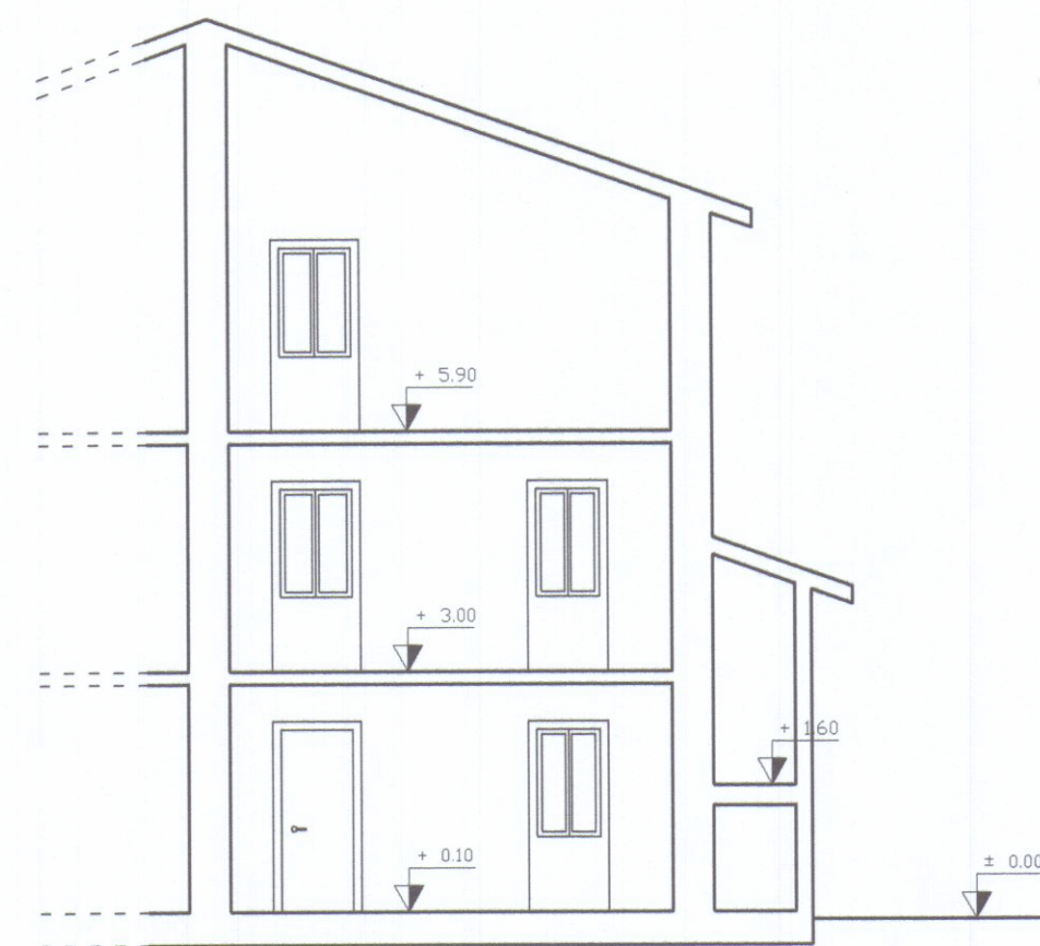
Sezione Y - Y¹
