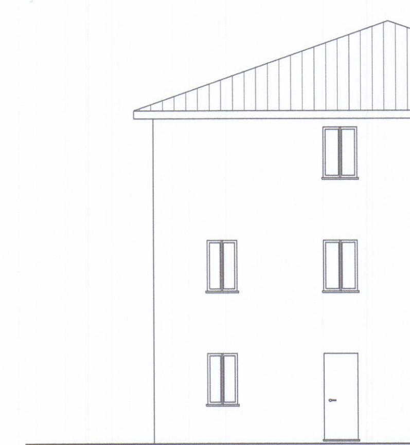
Prospetto lato Sud
