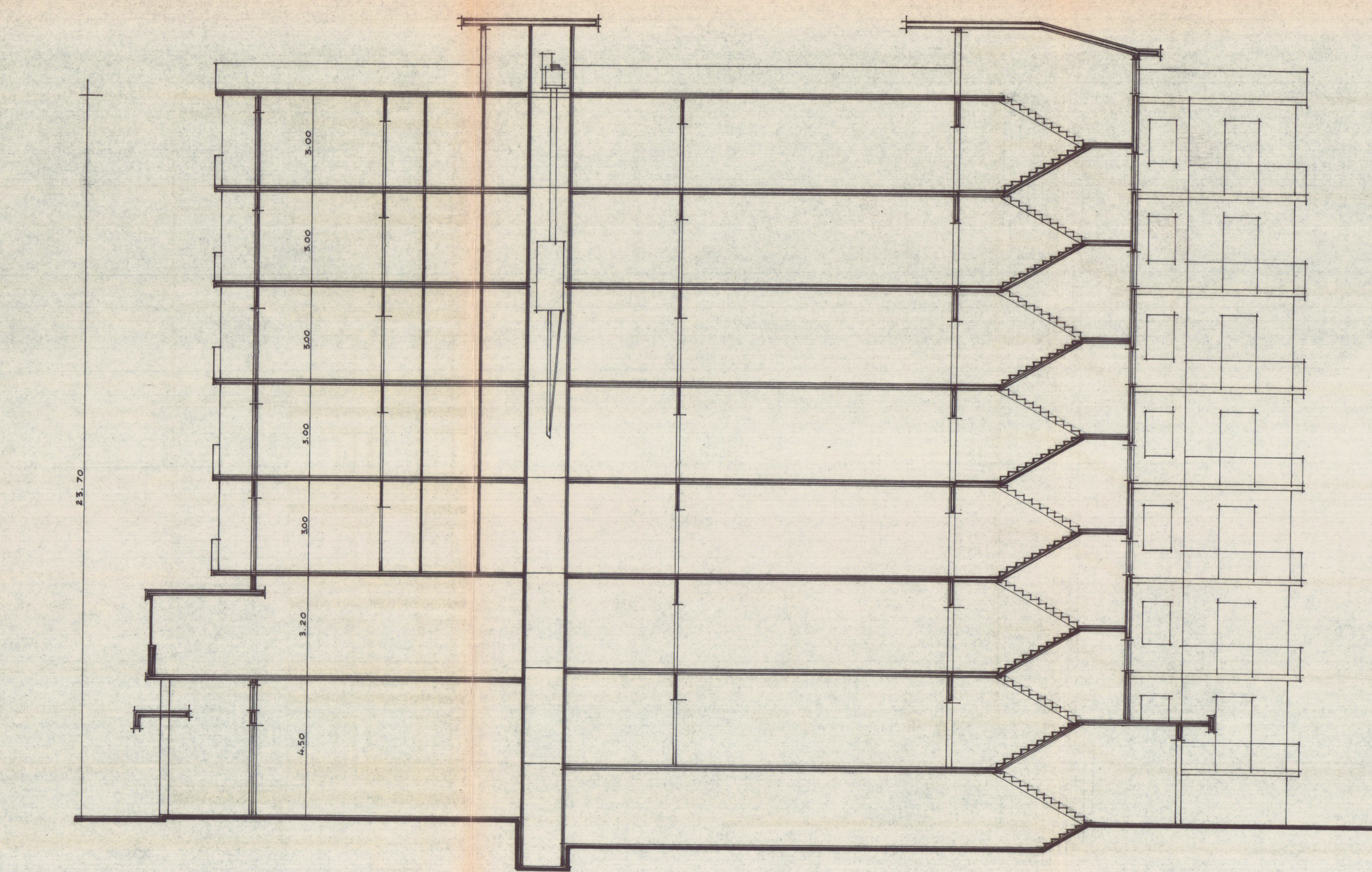
SEZIONE
