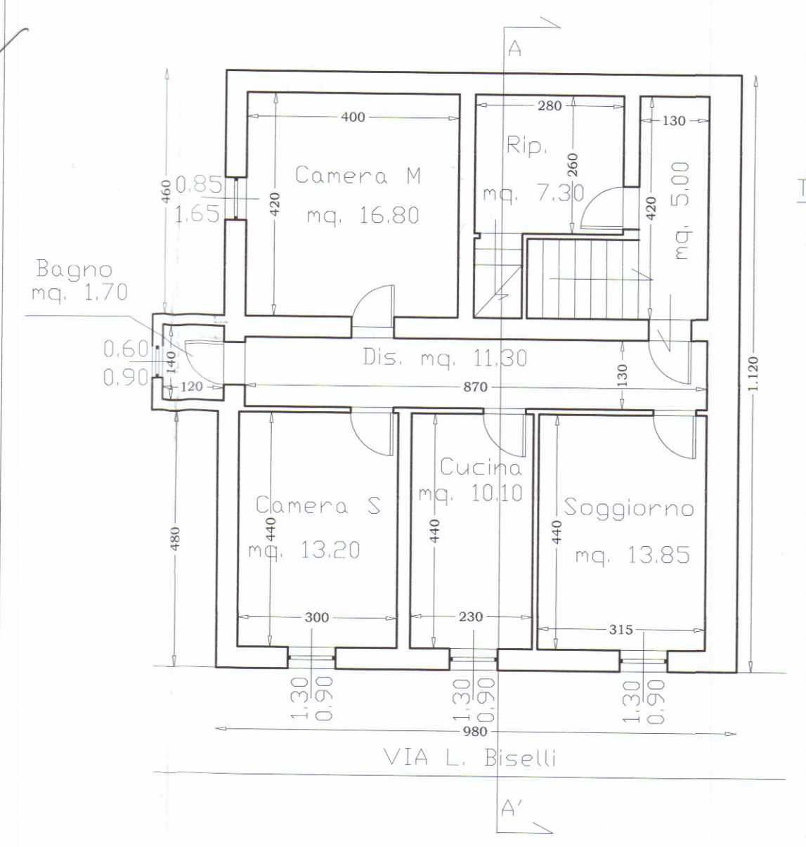
Pianta Piano Terzo
