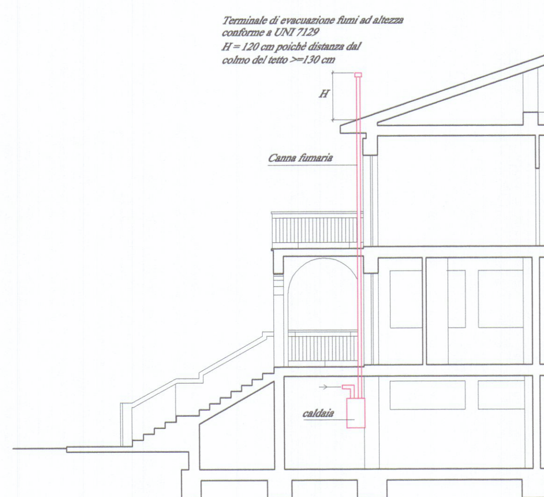
SEZIONE A-A
