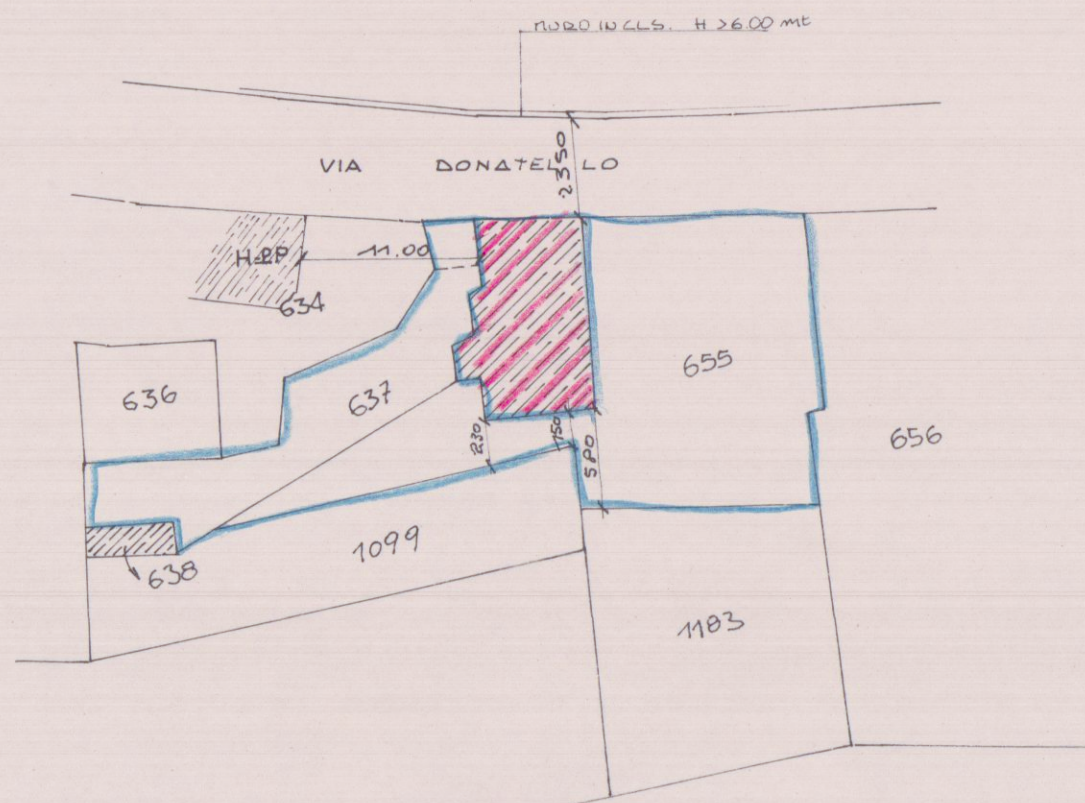
STRALCIO PLANIMETRICO 1:500
