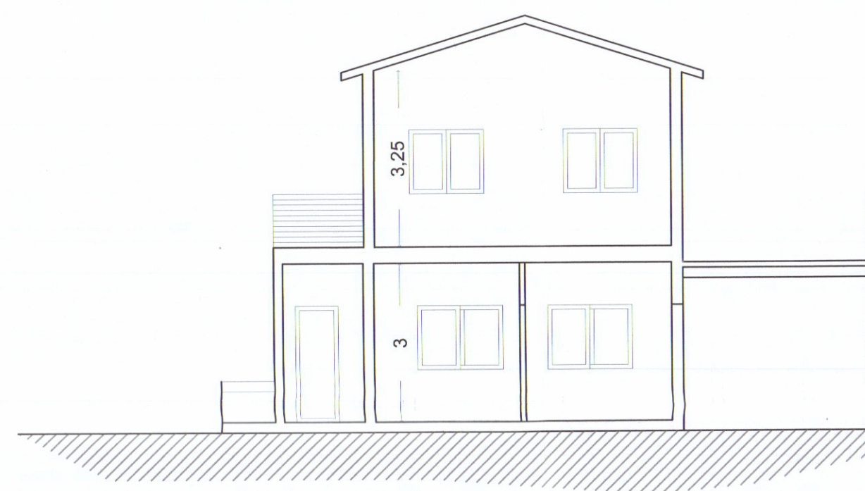
SEZIONE B-B
