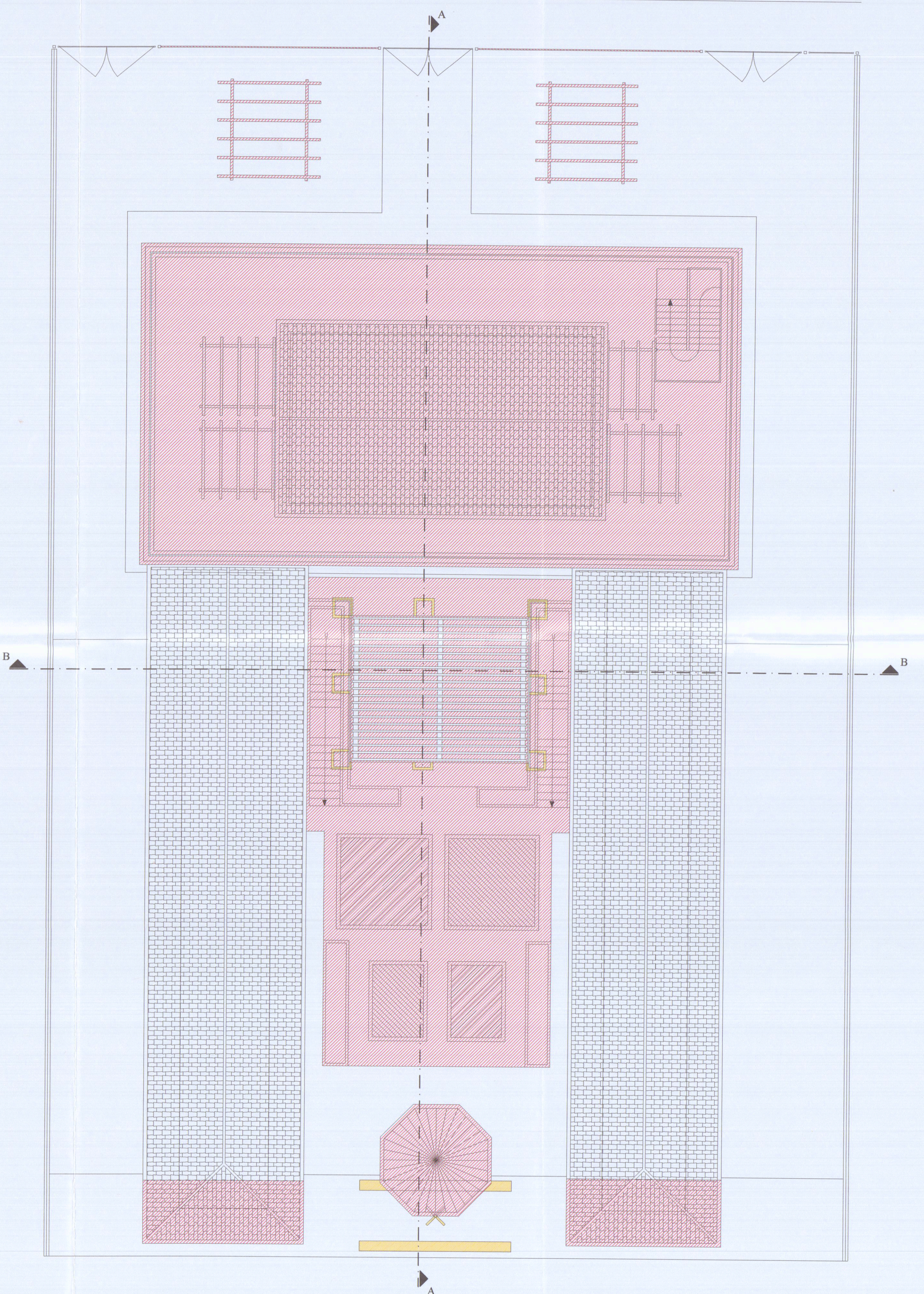
PIANTA COPERTURA
