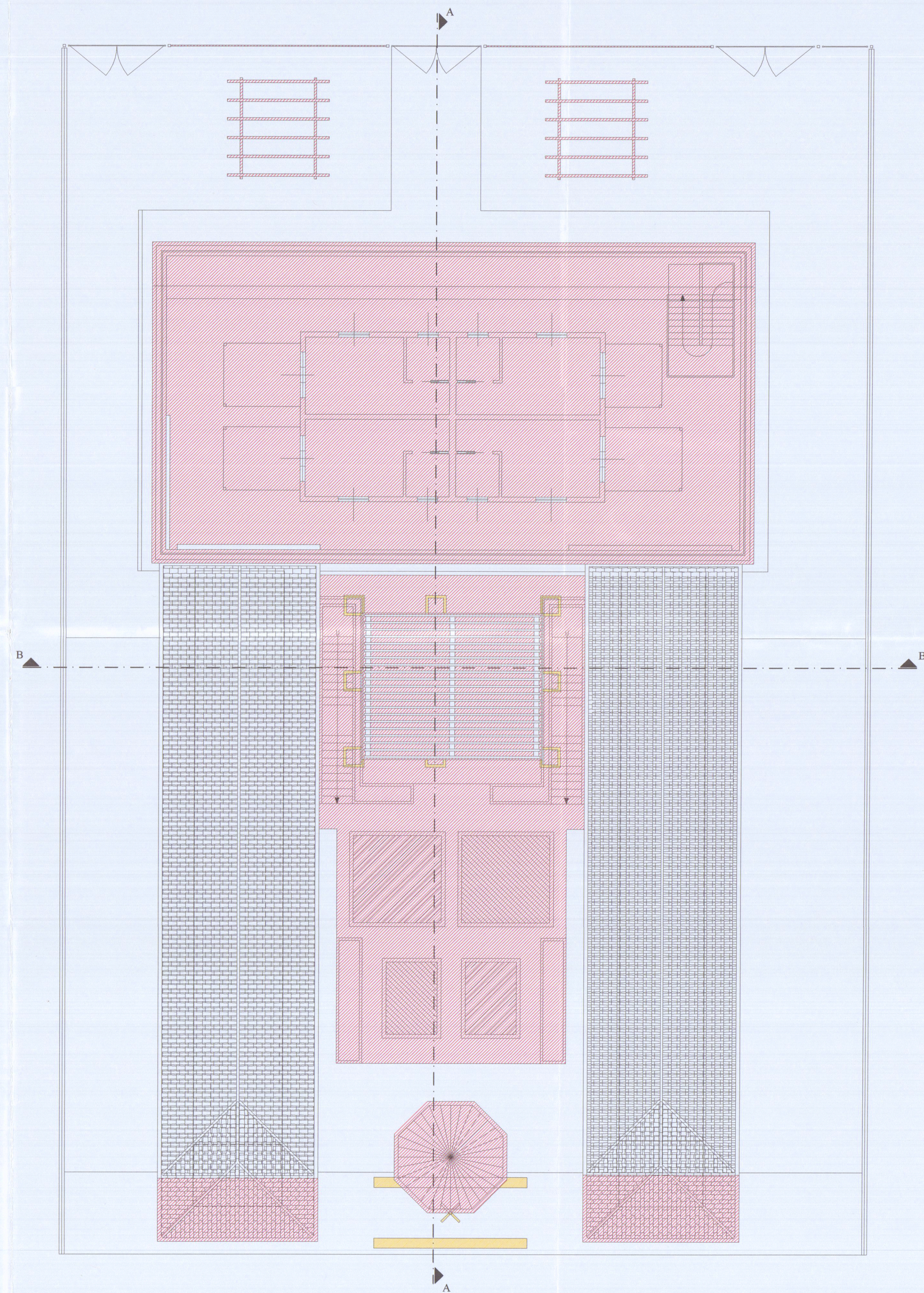
PIANTA PIANO PRIMO
