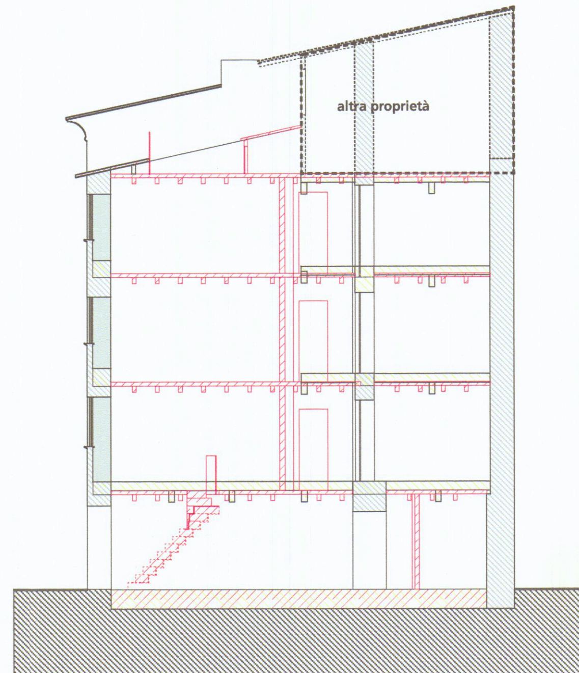
6 sezione scala 1: 100
