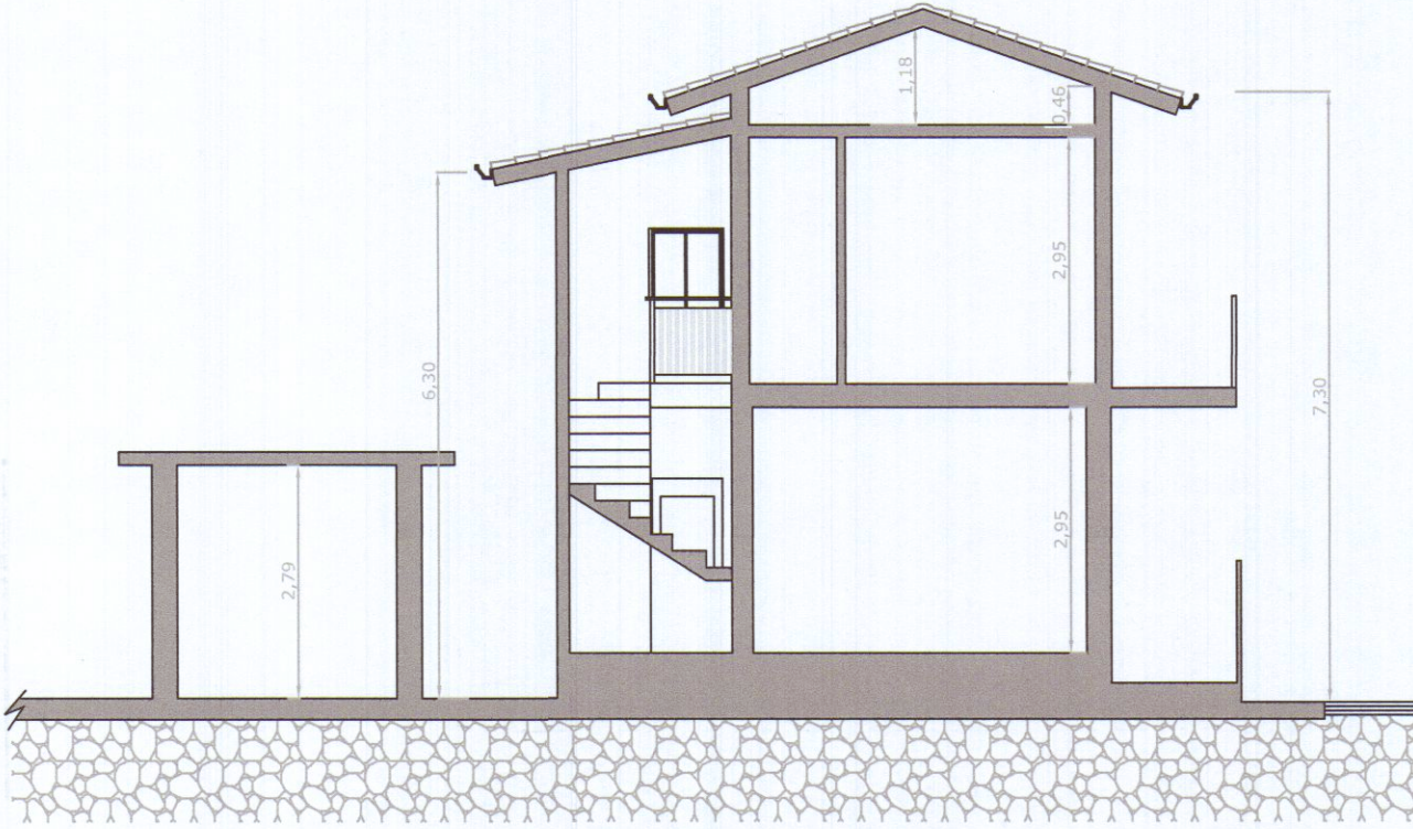
SEZIONE C-C
