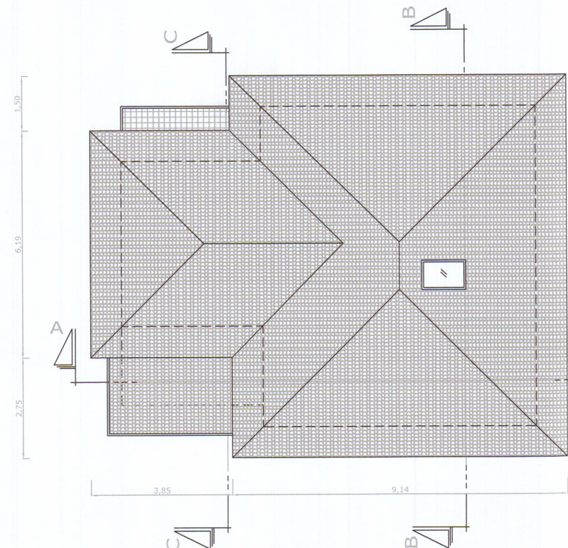
PIANO COPERTURA
