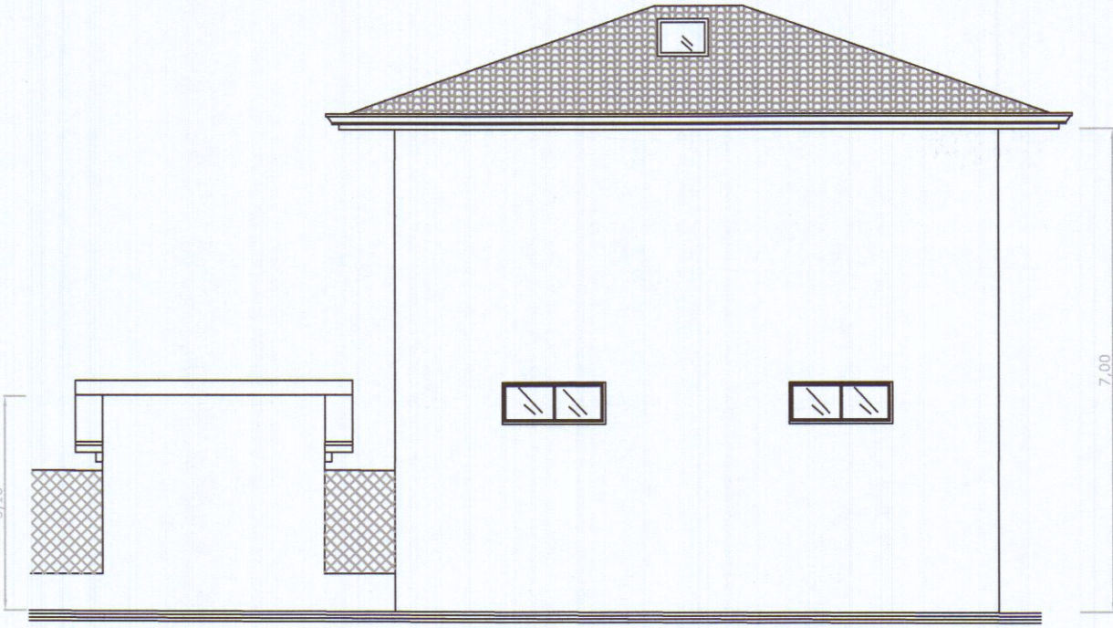
PROSPETTO OVEST
