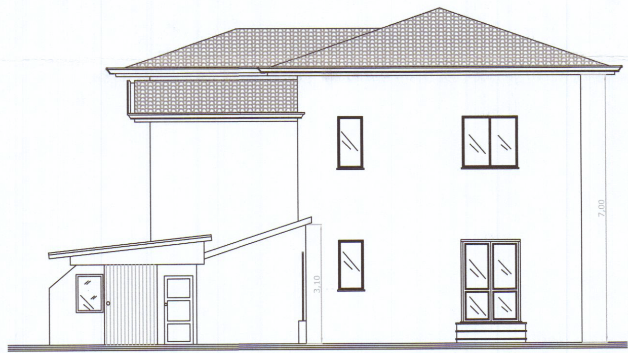
PROSPETTO NORD
