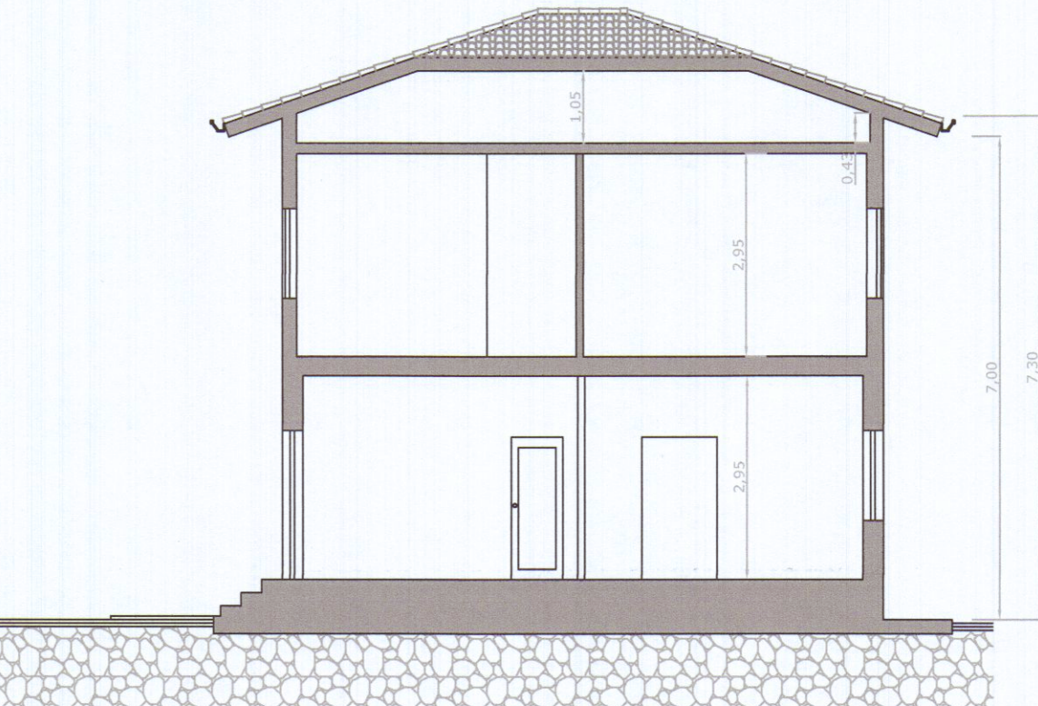
SEZIONE B-B
